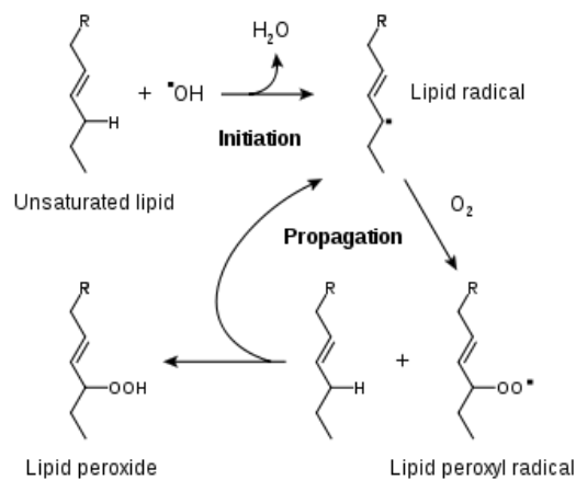
Schéma : mécanisme de peroxydation lipidique
