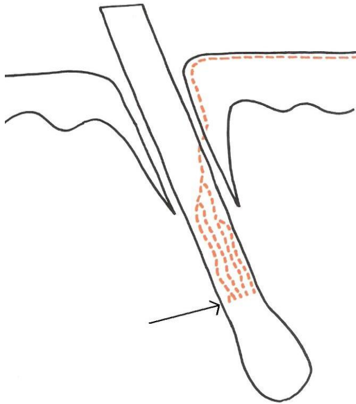
Figure 4 : Frange d'Adamson (1)
