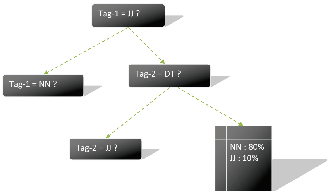
Figure 3 : Un simple arbre de décision
