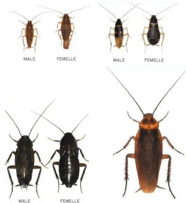
Figure 7 : les blattes domestiques en France, photos en taille réelle, avec de gauche à droite, en haut Blatella germanica et Supella longipalpa , en bas Blatta orientalis et Periplaneta americana (Source : http://www.ecolab-pest-france.fr )
