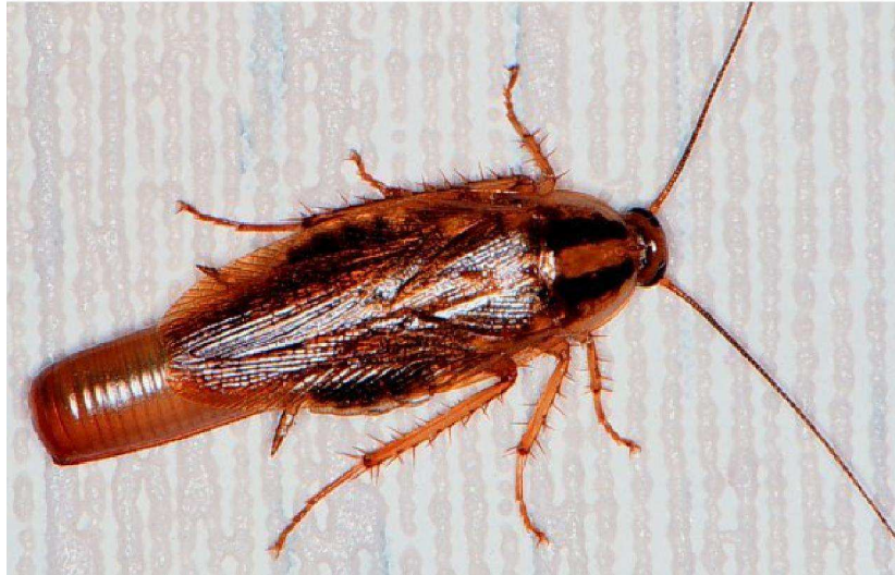
Figure 13 : Blatella germanica femelle porteuse d'une oothèque (31) (Source : ©University of Nebraska)
