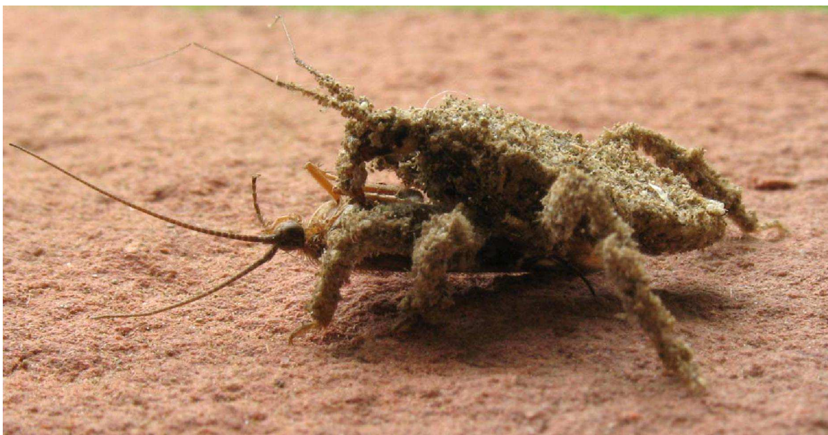
Figure 37 : Larve de réduve masquée couverte de poussière (98) (Source : ©andré lequet, http://www.insectes-net.fr/index.htm )
