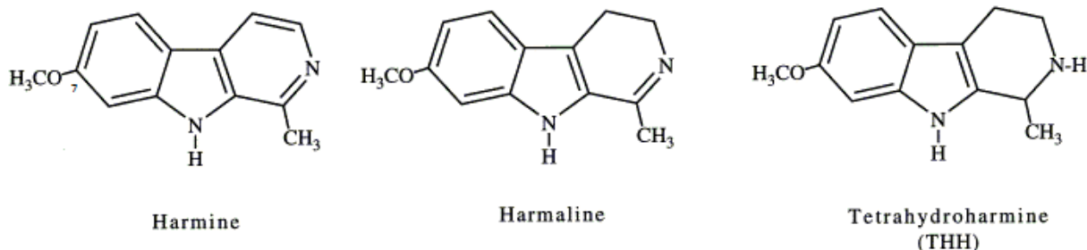
Figure 17: Principales \beta -carbolines de l'Ayahuasca
