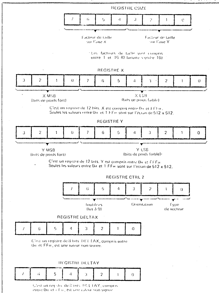
Fig. 1 - Constitution des différents registres pour l'écriture des caractères (taille, orientation et emplacement) et des vecteurs (registres DELTAX et DELTAY donnant leur projection)
