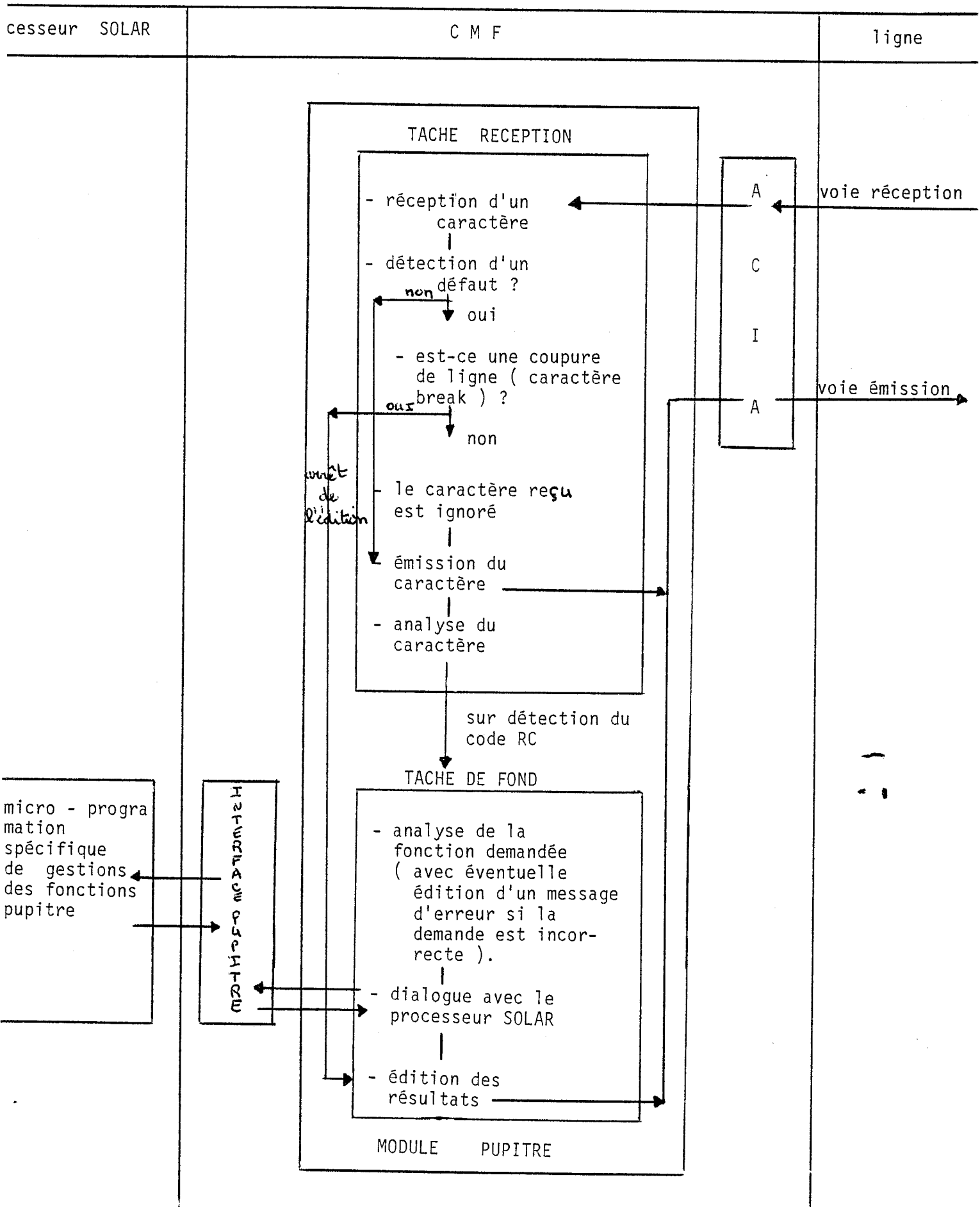
Figure IV.3 : Module pupitre
