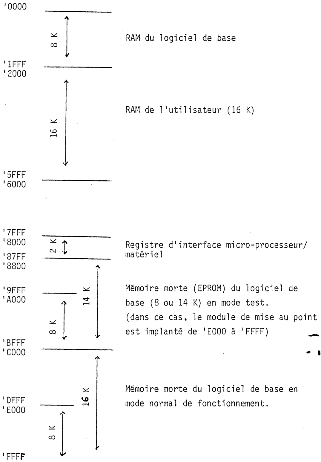
Figure 2.9. : espace d'adressage de µP1 si l'utilisateur utilise la mémoire vive seule.
