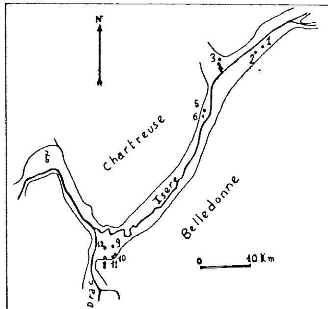
Fig.9— Localisation des échantillons (Aprahamian et al 1970)
