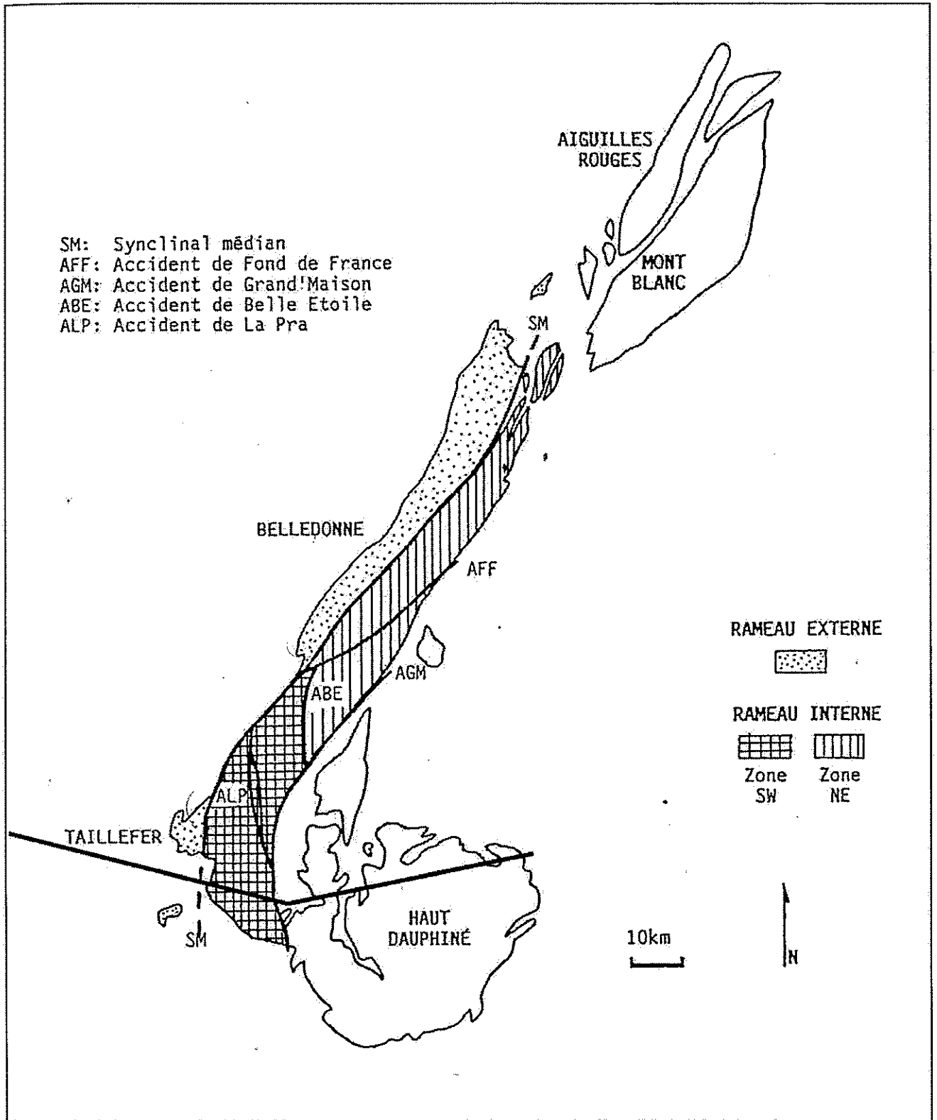
Figure I-3 : Schéma structural de la chaîne de Belledonne [Vivier et al. , 1987]. Le trait noir situe la coupe de la figure III-12a.
