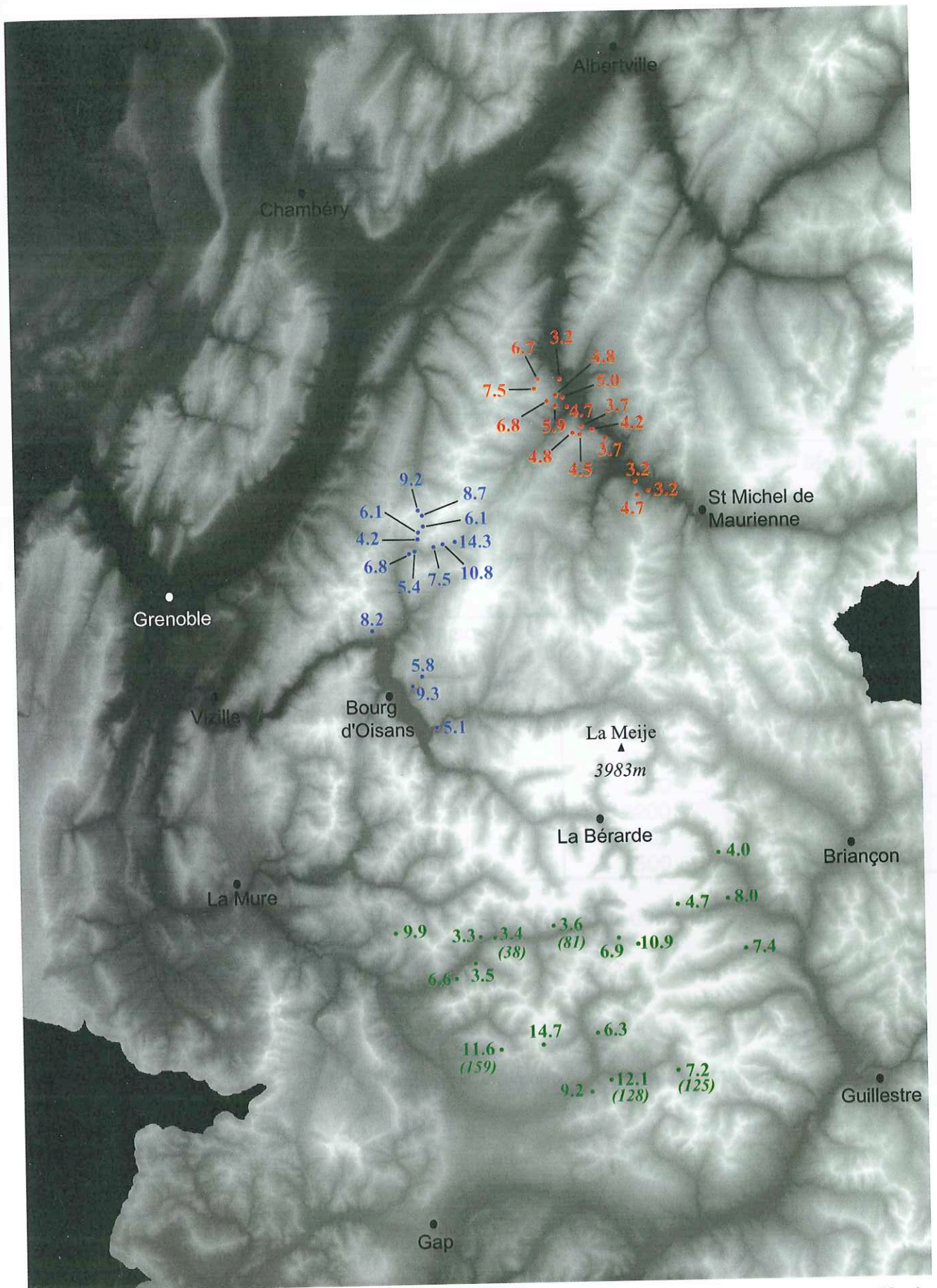
Figure II-6: Ages apparents TF en Ma obtenus sur apatite et sur zircon (italique) dans les massifs de Belledonne et du Pelvoux d'après les résultats de Lelarge (en rouge) en 1993, de Sabil (bleu) en 1995 et de Seward et al. (vert) en 1999.
