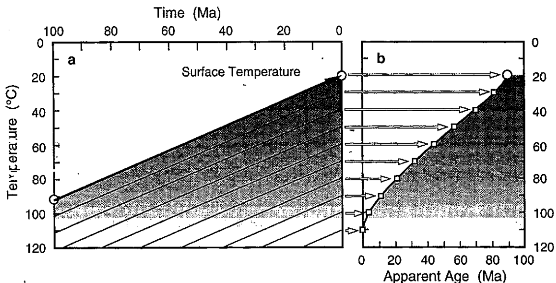
Figure II-4 : Modélisation du profil des âges traces de fission résultant d'un refroidissement régulier dans le temps de la croûte continentale [Gleadow & Brown, 2000].
