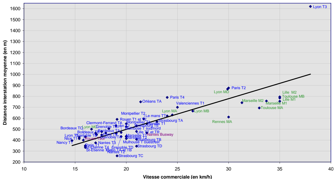
Figure 21 : Les vitesses commerciales moyennes en fonction des distances interstations
