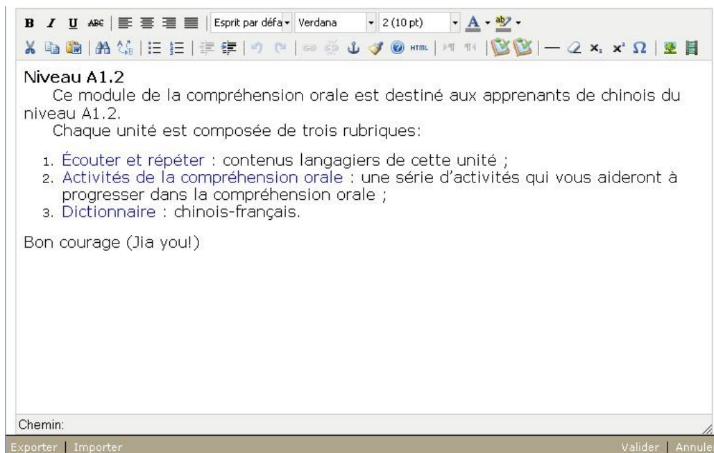
Figure 24: Texte formaté.
