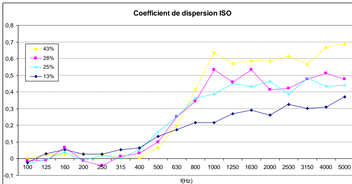
Fig. 39 – Coefficient de dispersion ISO du diffuseur hémisphérique de diamètre 20 cm, [SCHM 2005]. Le recouvrement du plan diffuseur par les demi-sphères est varié de 13 à 43 %. Le coefficient de dispersion ISO, après la fréquence de coupure du diffuseur à 400 Hz, augmente en fonction du pourcentage de recouvrement sur la plage considérée. Un effet de plateau est observé après 55 % environ.
