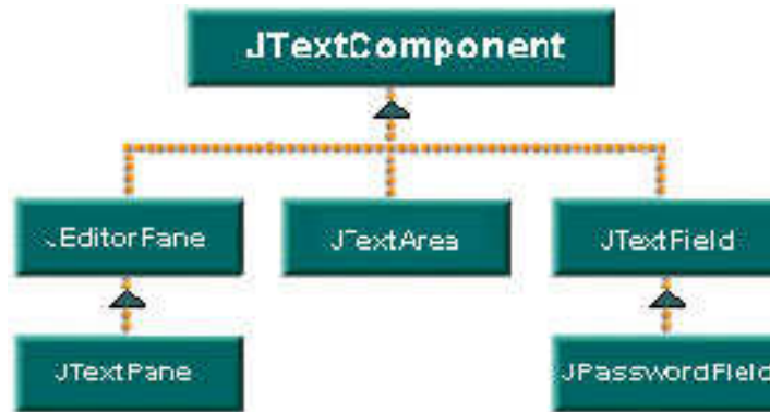
Figure 27 : Hiérarchie des classes Swing de textes Java
