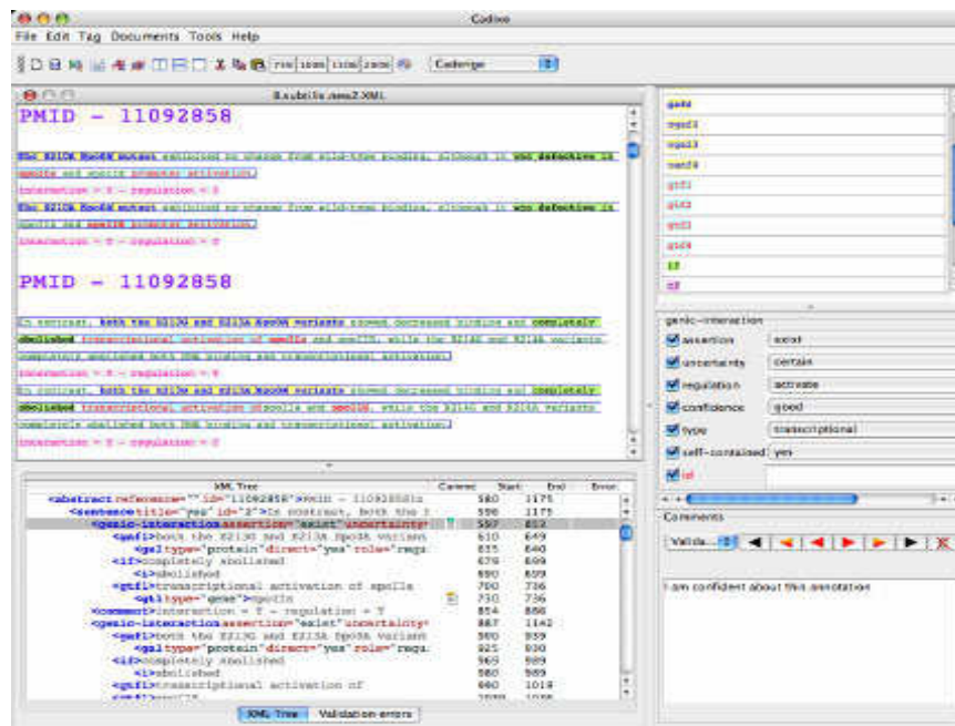
Figure 31 : Fenêtre principale de l'application CADIXE
