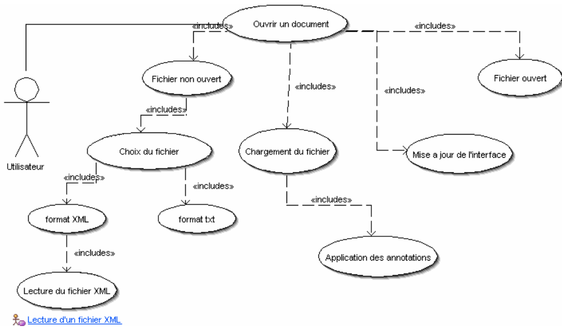
Figure 19 : Cas d'utilisation – Ouvrir un document
