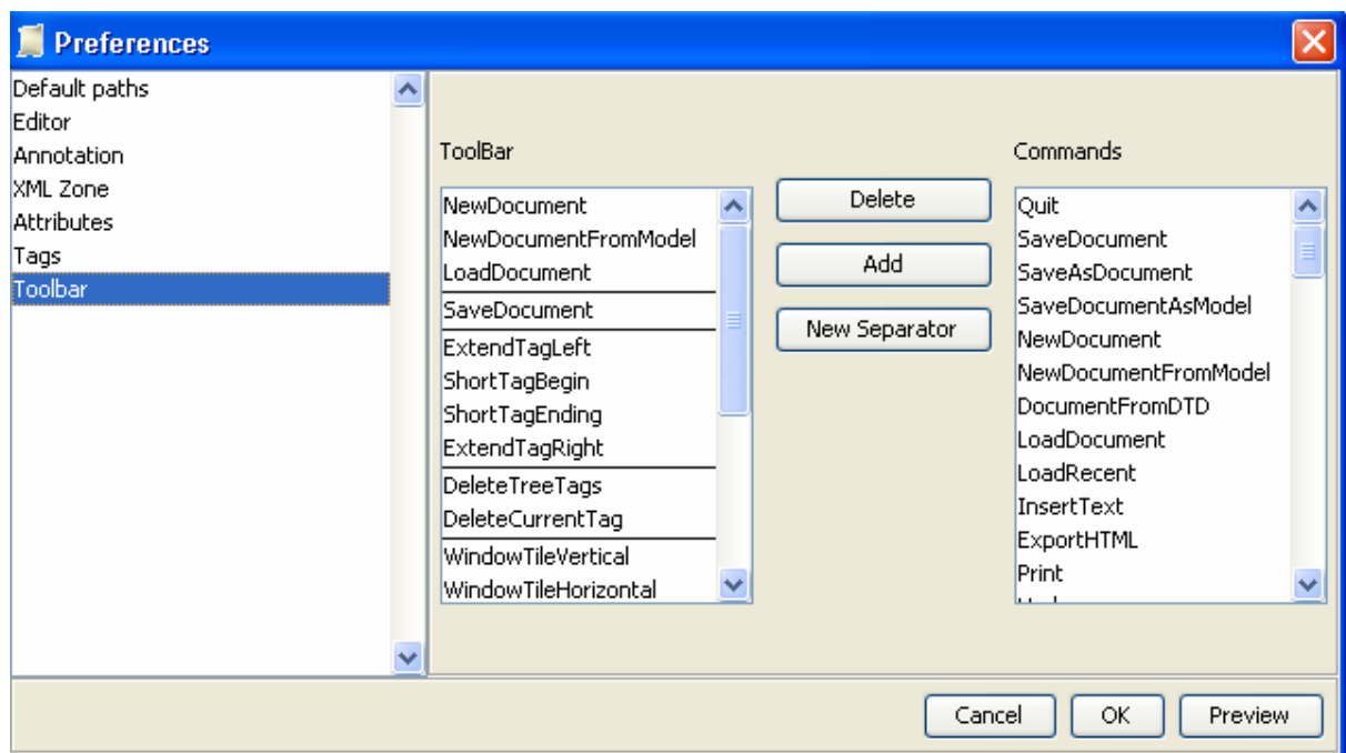
Figure 54 : Paramétrage des préférences « Toolbar »
