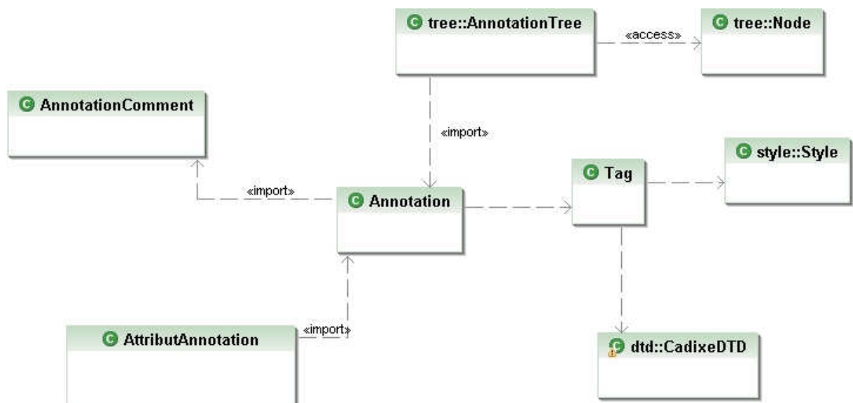
Figure 22: Associations entre certaines classes de l'application Cadixe
