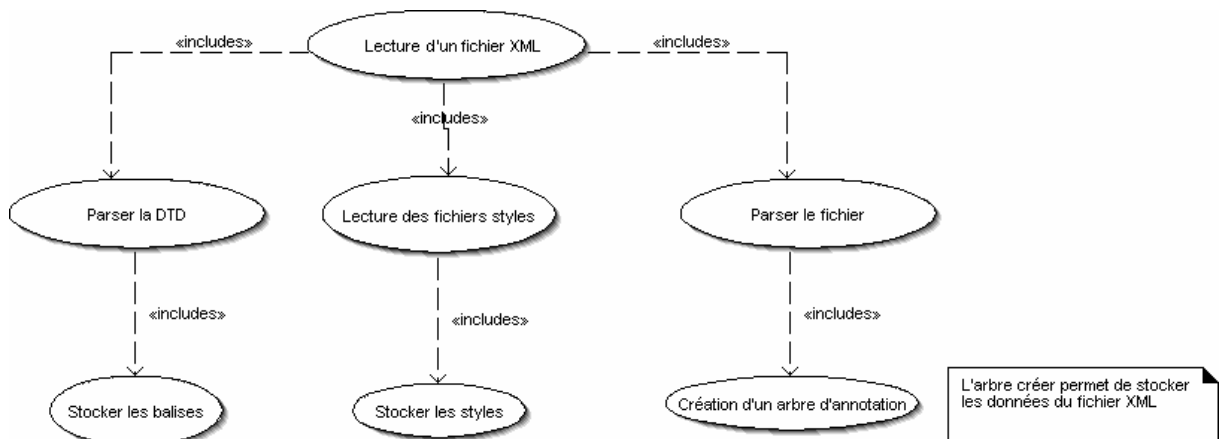
Figure 20 : Cas d'utilisation - Lecture d'un fichier XML
