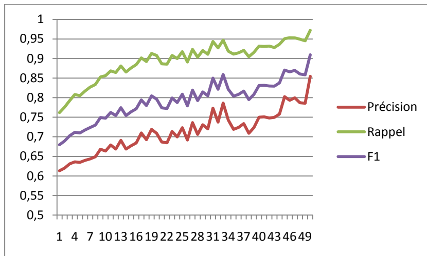
Figure 5 : résultats sur CORA, l'abscisse indique la taille des paquets
