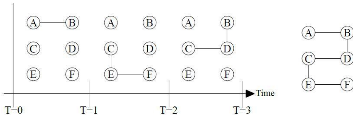
Figure 4 : exemple de graphe temporel à gauche et son résumé à droite (Tang, 2009)
