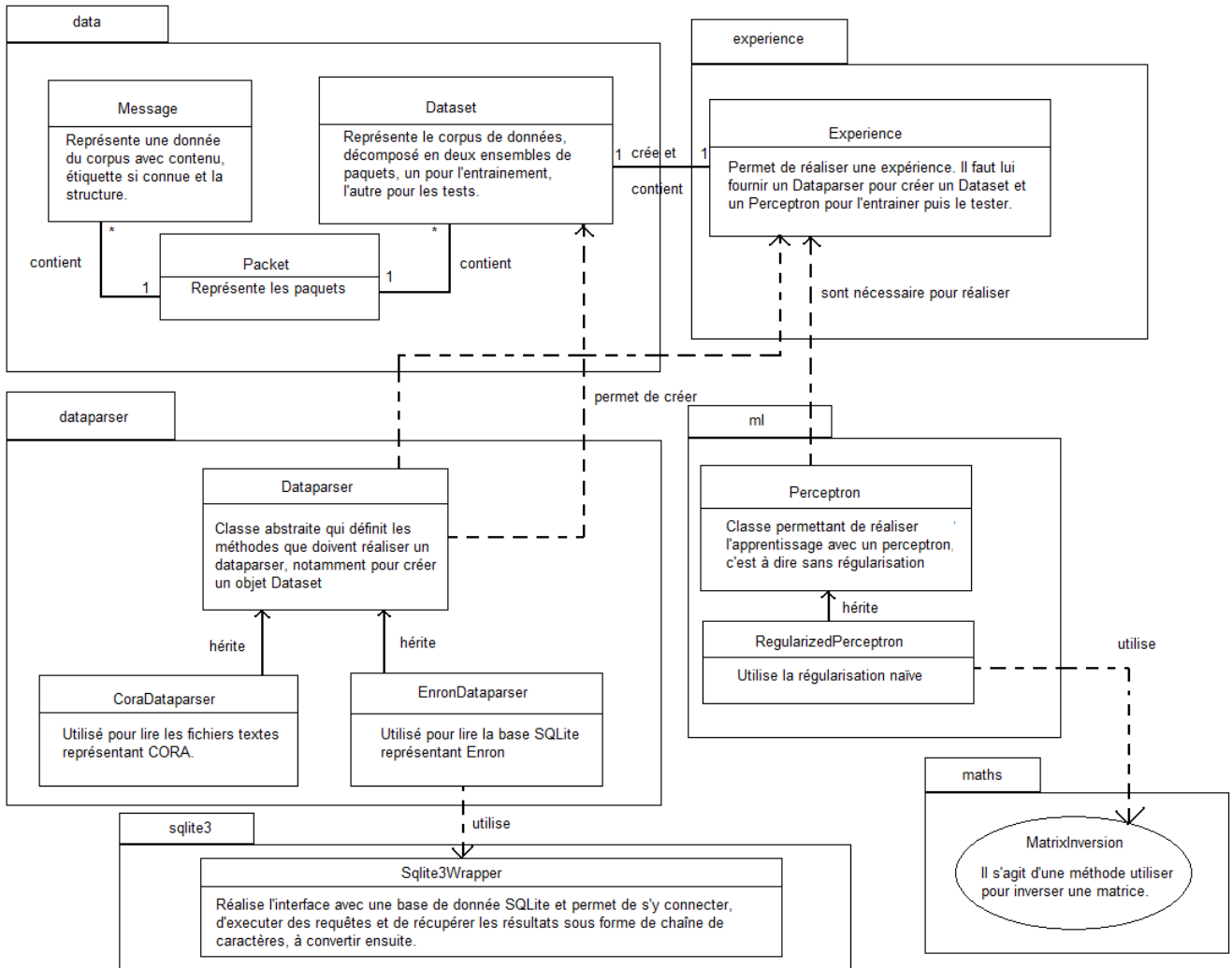
Figure 6 : pseudo-UML de la plateforme développée au cours de mon stage
