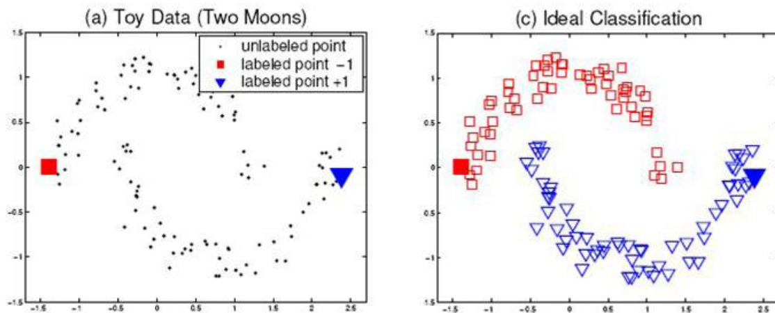
Figure 3 : le problème des deux lunes, extrait de (Zhou, 2004)
