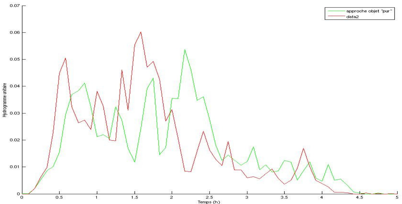
Fig.39 : Fonction de transfert de l’approche mixte et objet « pur » appliquées sur le bassin versant de la Chézine
