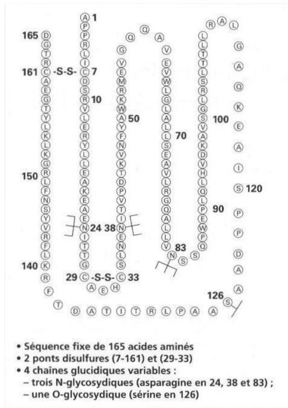
Figure 3 : Structure chimique de l'EPO 57
