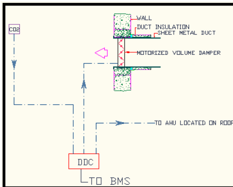
Figure VII-17: Diagramme de contrôle des vannes d'apport d'air
