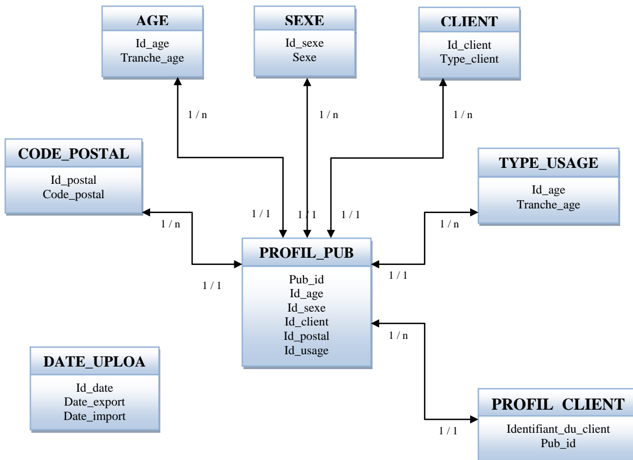
Modèle conceptuel des données de la plateforme de calcul des profils publicitaires
