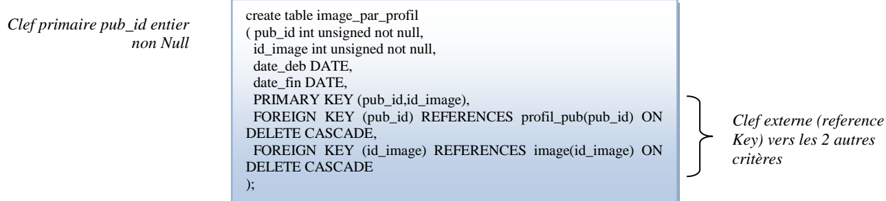
Code SQL de l'association des images à un profil publicitaire
