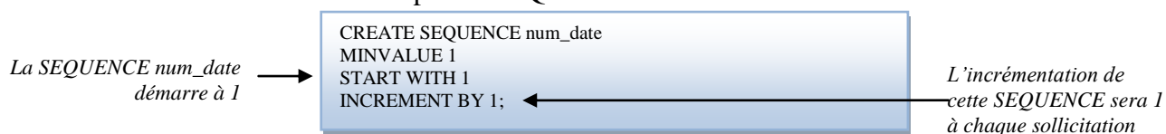
Code SQL de la création d'une SEQUENCE Oracle
