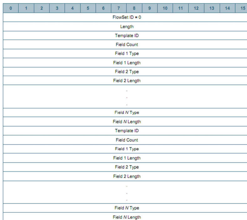
Figure 35 : Format du Template FlowSet des trames NetFlow d'export version 9 (Cisco Systems, 2007a)
