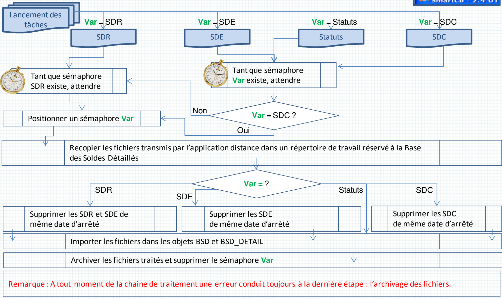
Figure 14 - Algorithme d'acquisition des flux de la BSD
