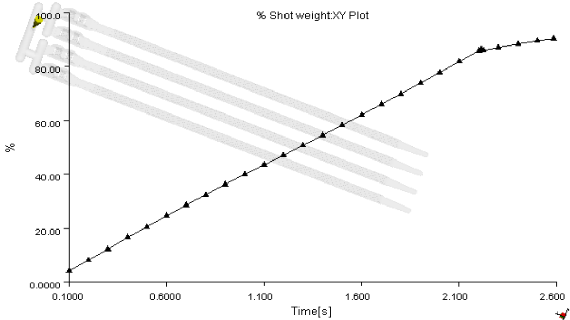
Figure 36g : Simulation de l'évolution de remplissage en % dans colliers de serrage
