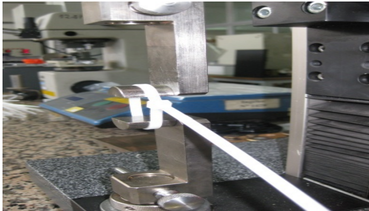
Figure 25 : Photo de la machine de traction de la boucle
