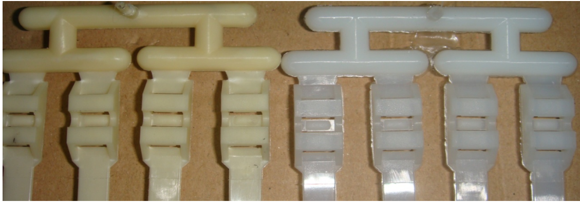
Figure 59: Comparaison entre 2 moulées à gauche PA/PP et à droite en PA66
