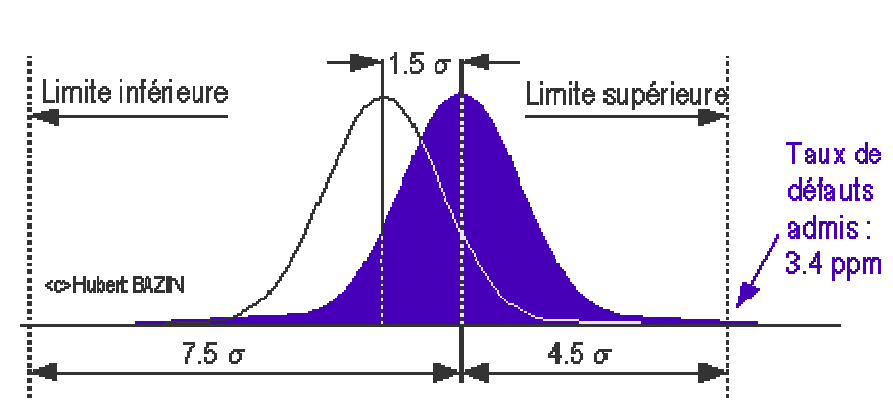
Figure 5: Comportement d'un procédé placé sous contrôle 6σ avec un décentrage de 1,5\sigma [31]
