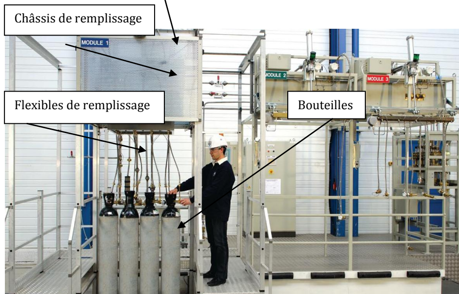
Photo d'une rampe de remplissage Cryostar®
