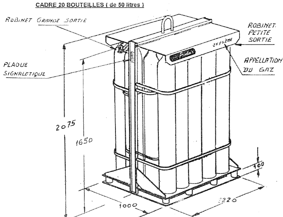
Figure 7: Cadre 20 bouteilles
