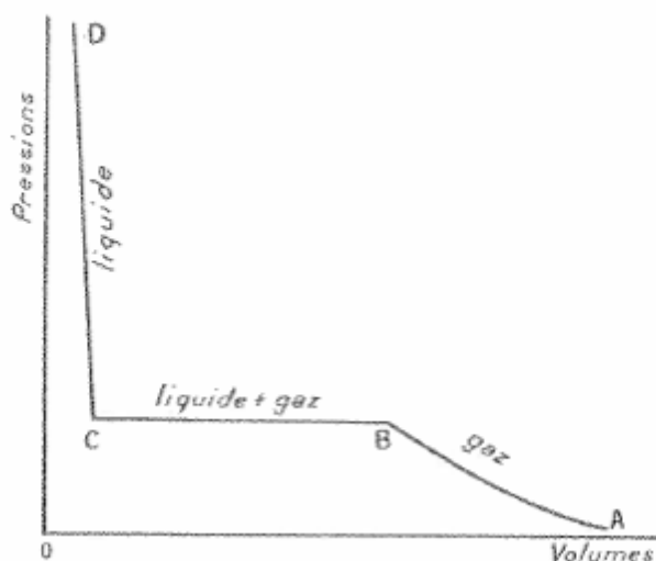
Figure 2: Evolution des volumes en fonction de la pression
