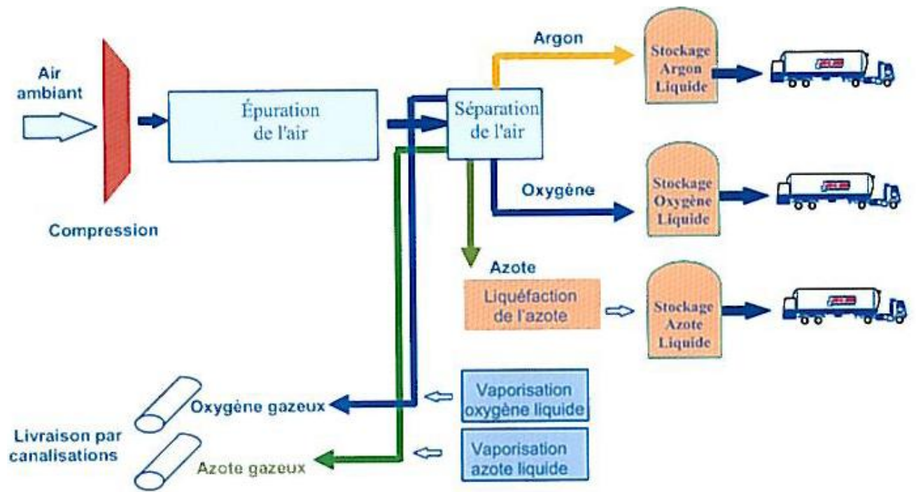
Figure 12: Schéma de processus d'obtention d'oxygène, d'argon et d'azote
