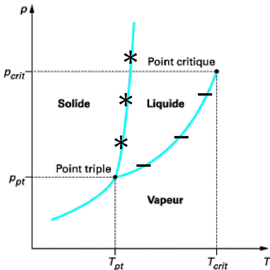
Figure 1: Diagramme de phase (pression-température)
