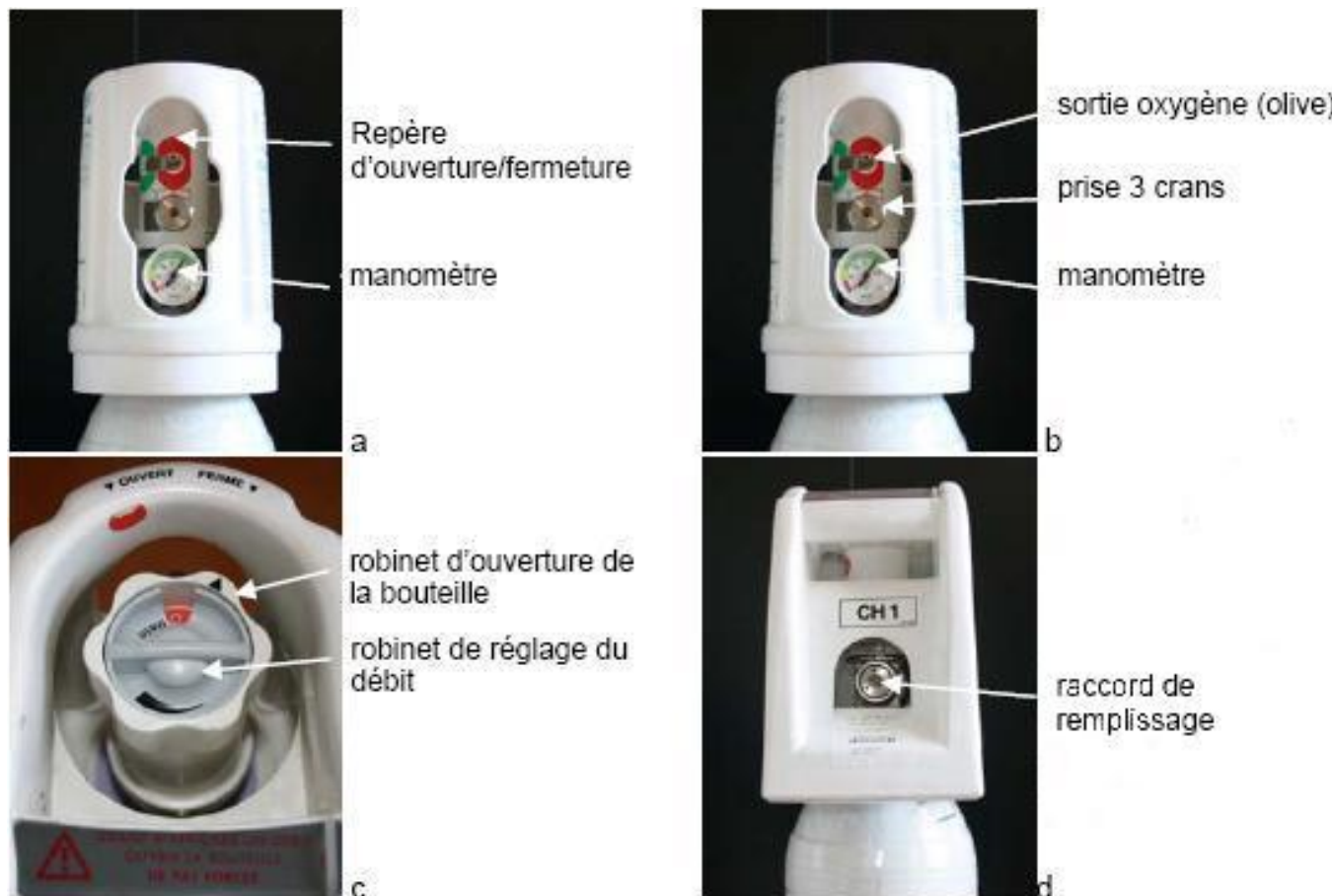
Figure 6: éléments du chapeau d'une bouteille de gaz
