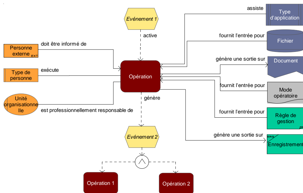
Figure 24 : symboles du modèle CPEe
