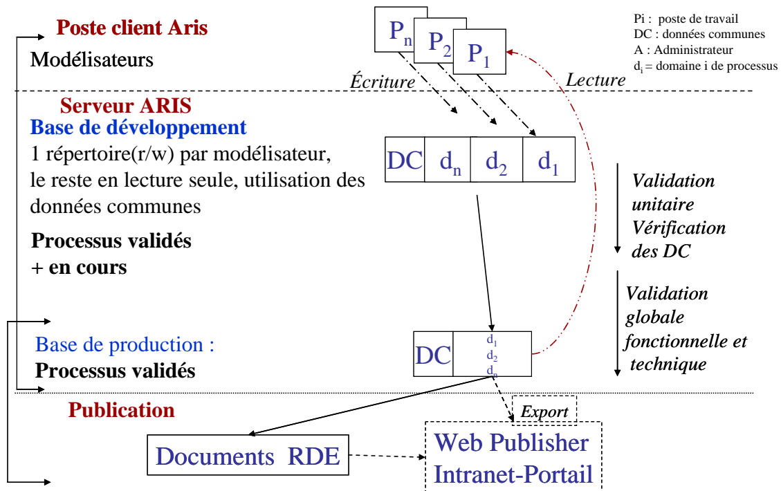
Figure 29 : flux de l'environnement de modélisation
