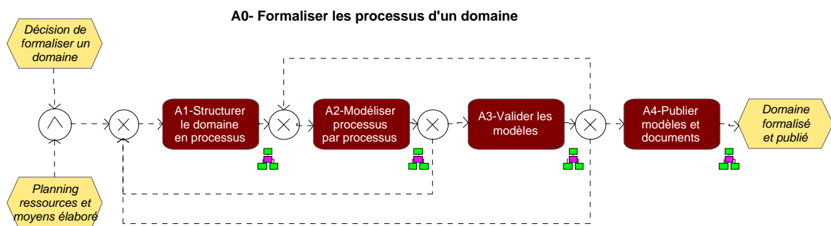
Figure 16 : processus formaliser un processus
