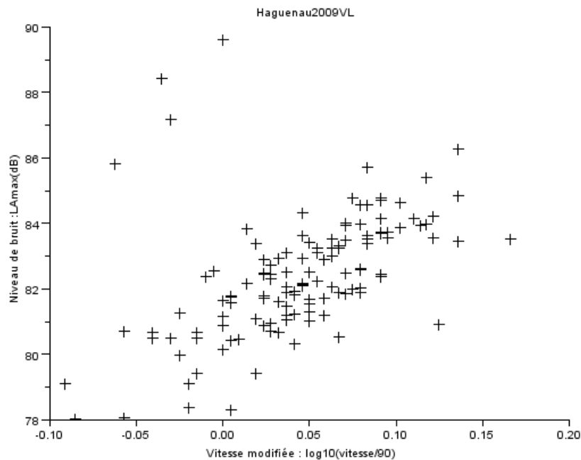
FIGURE 2.1 – Un jeu de données
