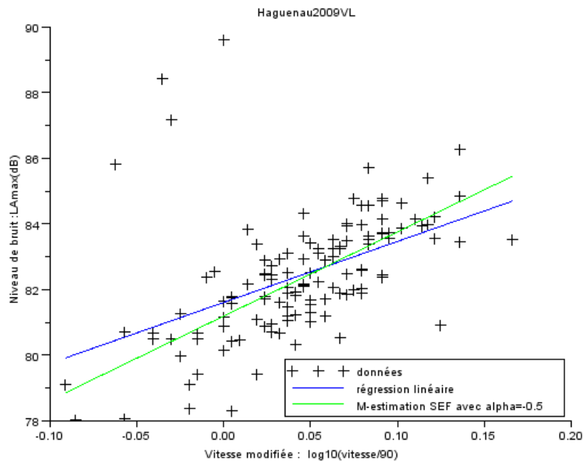
FIGURE 2.6 – Droite obtenue par M-estimation (SEF \alpha = -0.5 )
