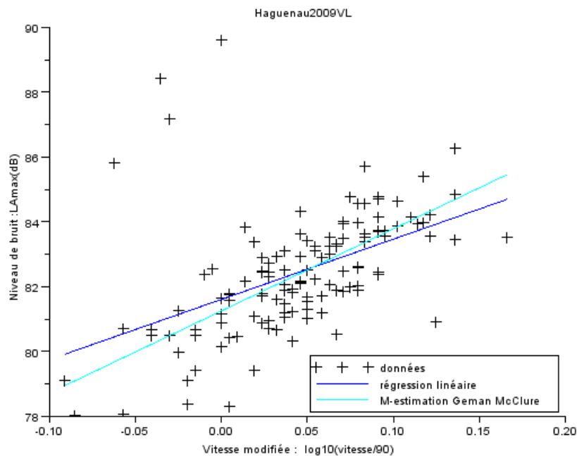
FIGURE 2.3 – Droite obtenue par M-estimation (Geman et McClure)
