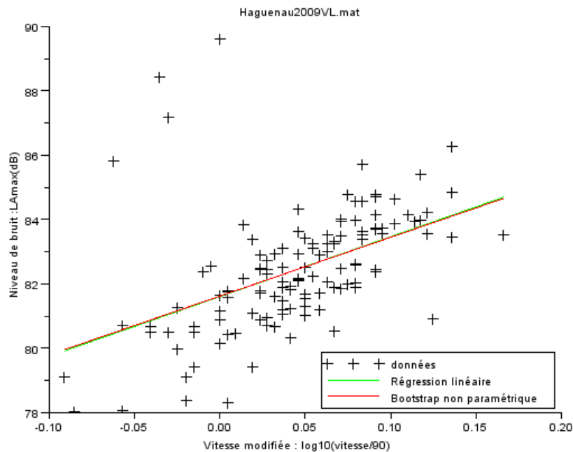
FIGURE 5.1 – Comparaison - droite issue de régression linéaire et droite issue du bootstrap non paramétrique, suivi de régression linéaire
