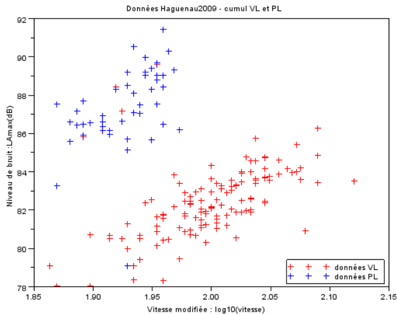
FIGURE 4.1 – Haguenau2009 : Superposition de données VL et PL
