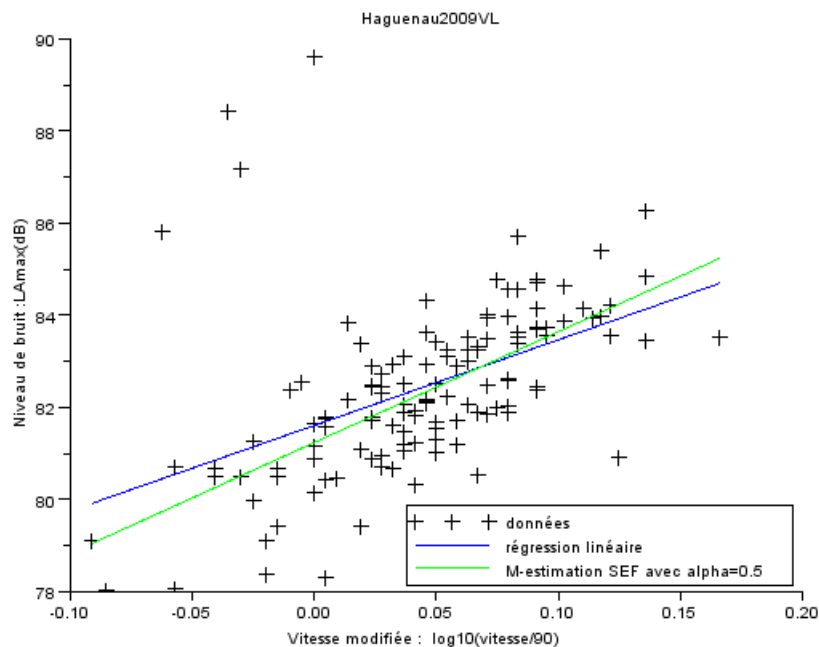
FIGURE 2.4 – Droite obtenue par M-estimation (SEF \alpha = 0.5 )
