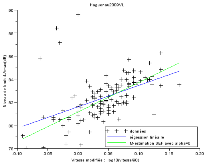
FIGURE 2.5 – Droite obtenue par M-estimation (SEF \alpha = 0 )
