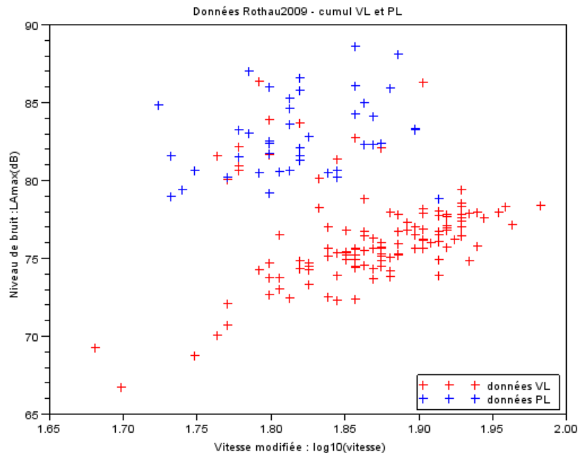
FIGURE 4.6 – Rothau2009 : Superposition de données VL et PL
