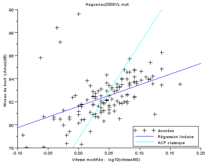
FIGURE 3.1 – Droite obtenue par ACP
