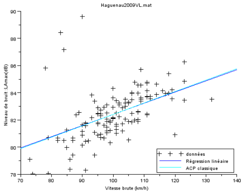
FIGURE 3.2 – Droite obtenue par ACP sur les vitesses brutes
