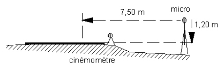
FIGURE 1.3 – Vue en travers
