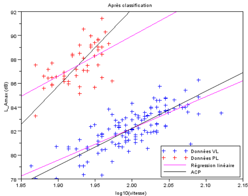
FIGURE 4.5 – Classification après l’algorithme
