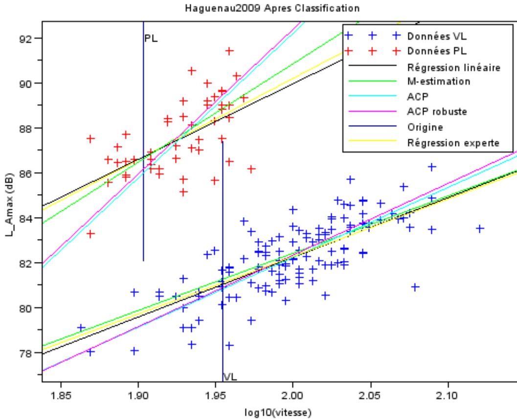
FIGURE 6.2 – Haguenau2009 : Résultats après classification
