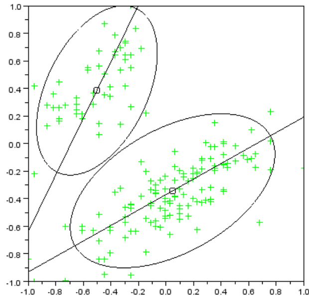
FIGURE 4.3 – Avant l’algorithme - initialisation avec deux lois normales
