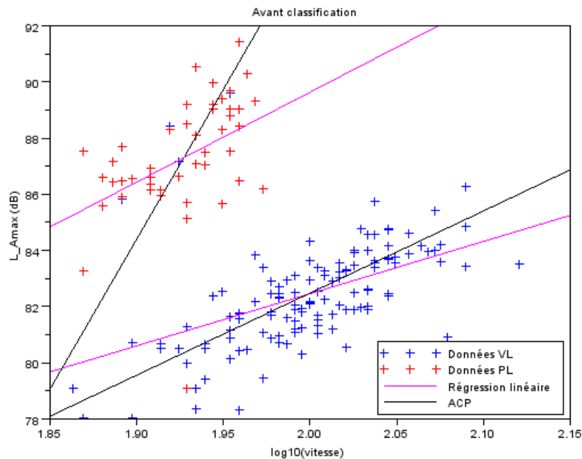
FIGURE 4.2 – Avant l’algorithme - droites ACP
