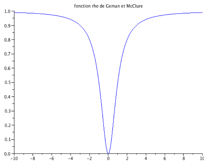
FIGURE A.1 – Geman et McClure
