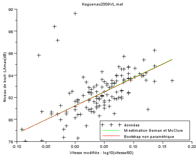
FIGURE 5.2 – Comparaison - droite issue de M-estimation et droite issue du bootstrap non paramétrique, suivi de M-estimation
