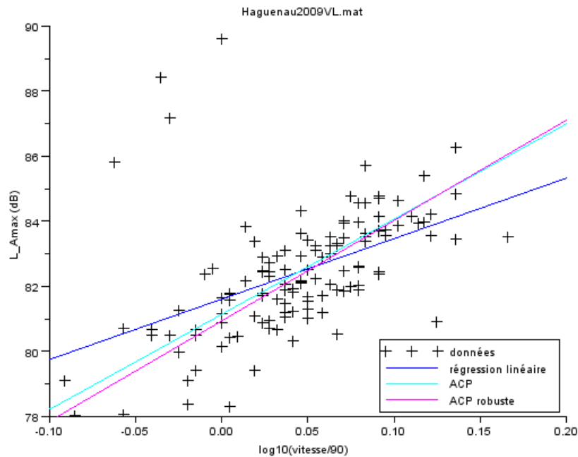
FIGURE 3.5 – Droites obtenues par ACP et ACP robuste
