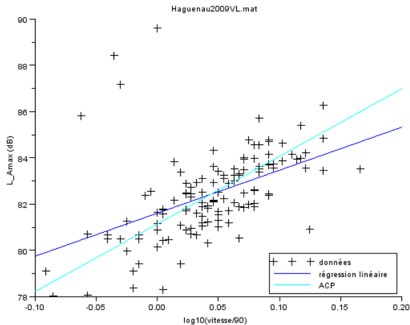
FIGURE 3.4 – Courbes obtenues par régression linéaire et ACP sur données normalisées
