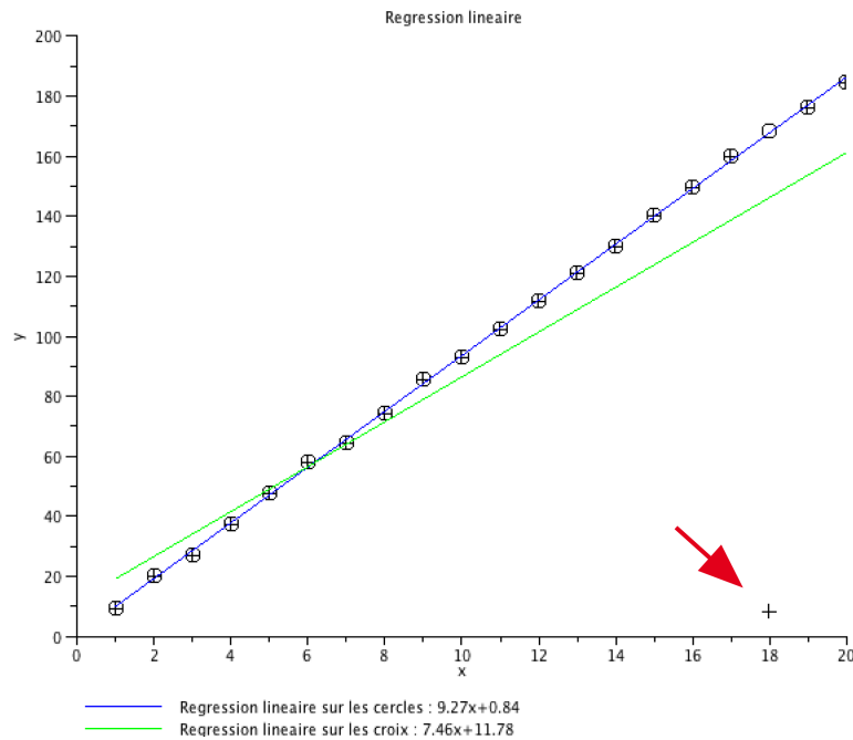
FIGURE A.3 – Droite des moindres carrés et point aberrant
