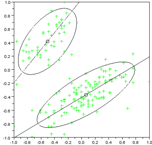
FIGURE 4.4 – Après l’algorithme - représentation des deux lois normales obtenues
