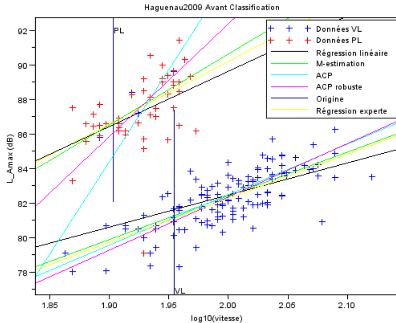
FIGURE 6.1 – Haguenau2009 : Résultats avant classification
