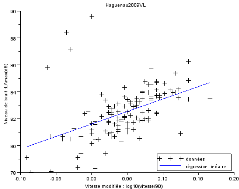
FIGURE 2.2 – Droite obtenue par régression linéaire
