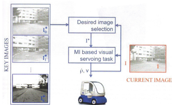
FIGURE 3.3 – Figure tirée de [10]. Boucle algorithmique de la navigation basée sur un asservissement visuel utilisant l'information mutuelle.
