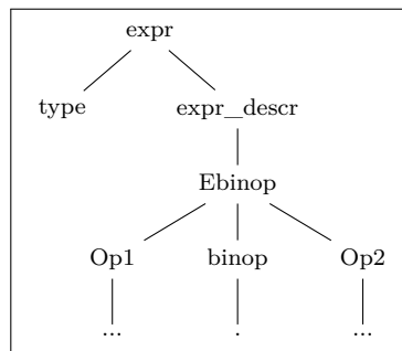
FIG. 5.4 – Arbre syntaxique de l'opération d'addition obfusqué
