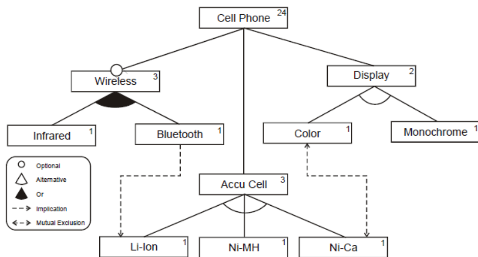
Figure 16. Exemple d'un diagramme de caractéristiques(33)
