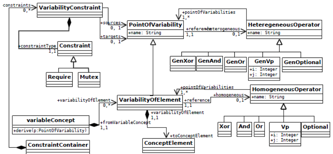
Figure 12. Méta-modèle variabilité Morin et al. (30)
