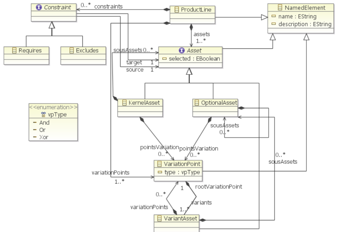
Figure 13. Méta modèle LdP proposé
