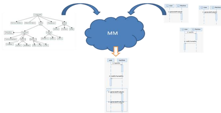
Figure 36. Méta-modèle Kermeta
