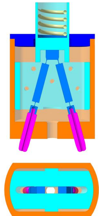
Figure 57 : Vue en coupe de face et de dessus du préhenseur.
