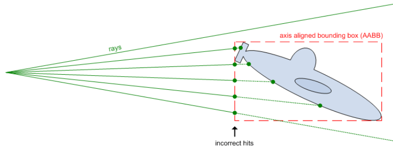
FIG. 6 – Lancer de rayons sur une boîte englobante alignée sur les axes. On peut remarquer l'apparition de rayons coupés qui ne devraient pas l'être. Image prise sur le site d'Ogre3D[2]
