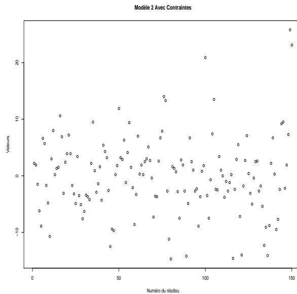
FIGURE 4.6: Residus Modèle 2
