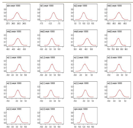
FIGURE 4.2: Densité des lois a posteriori
