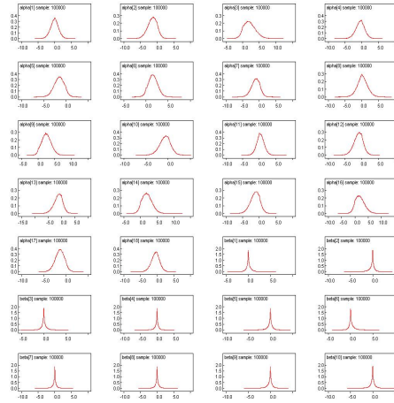
FIGURE 5.2: Densité des lois a posteriori
