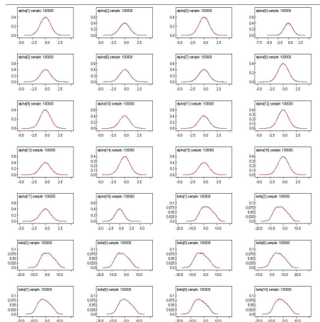
FIGURE 5.1: Densité des lois a posteriori
