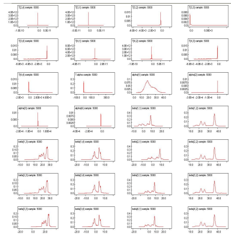
FIGURE 6.1: Densité du modèle mixte
