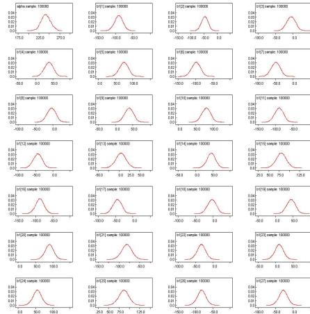
FIGURE 4.5: Densité des lois a posteriori
