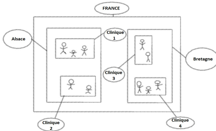
FIGURE 3.1: Exemple de Structure hiérarchique
