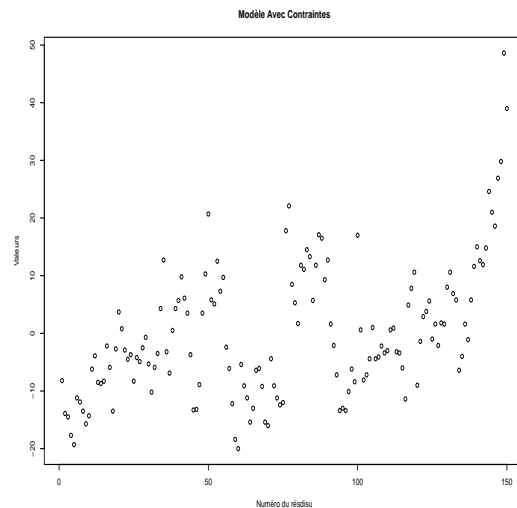
FIGURE 4.3: Résidus du modèle avec contrainte
