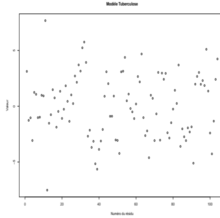
FIGURE 5.3: Résidus Modèle 1
