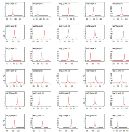
FIGURE 6.2: Densité du modèle mixte avec l'utilisation du n.thin
