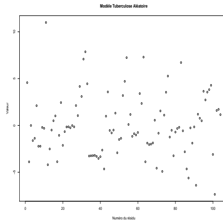
FIGURE 5.4: Résidus Modèle avec Sujet
