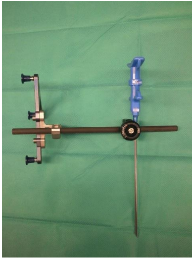
Montage sur trocart de vertébroplasties
