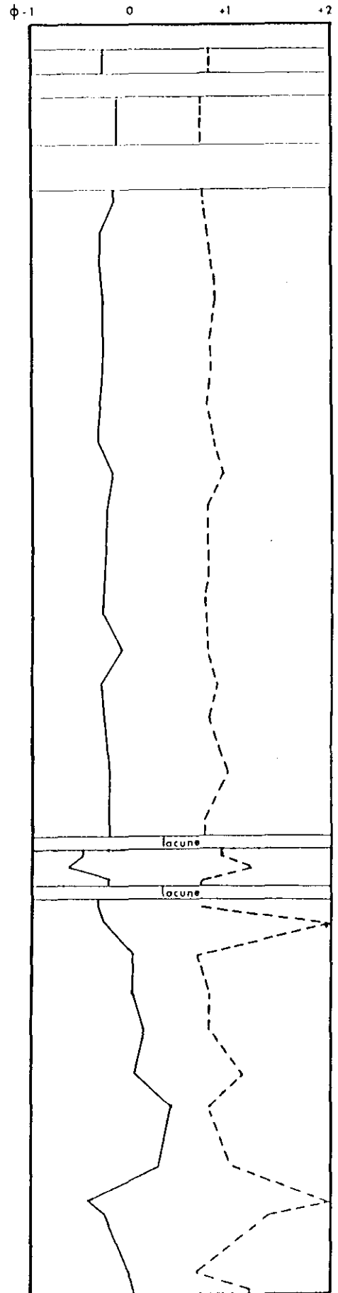
Fig. 16 - Coupes A, B et C. Evolution verticale des indices d'Assymétrie et d'Acuité.
