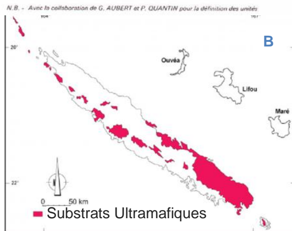
B : Localisation des substrats ultrabasiqes, jso.revues.org
