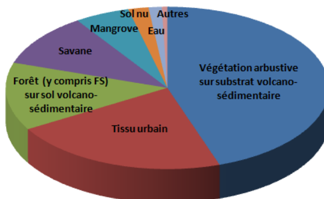
Fig. 12 : Répartition des types d'occupation des sols de l'UPF1 en 2008
