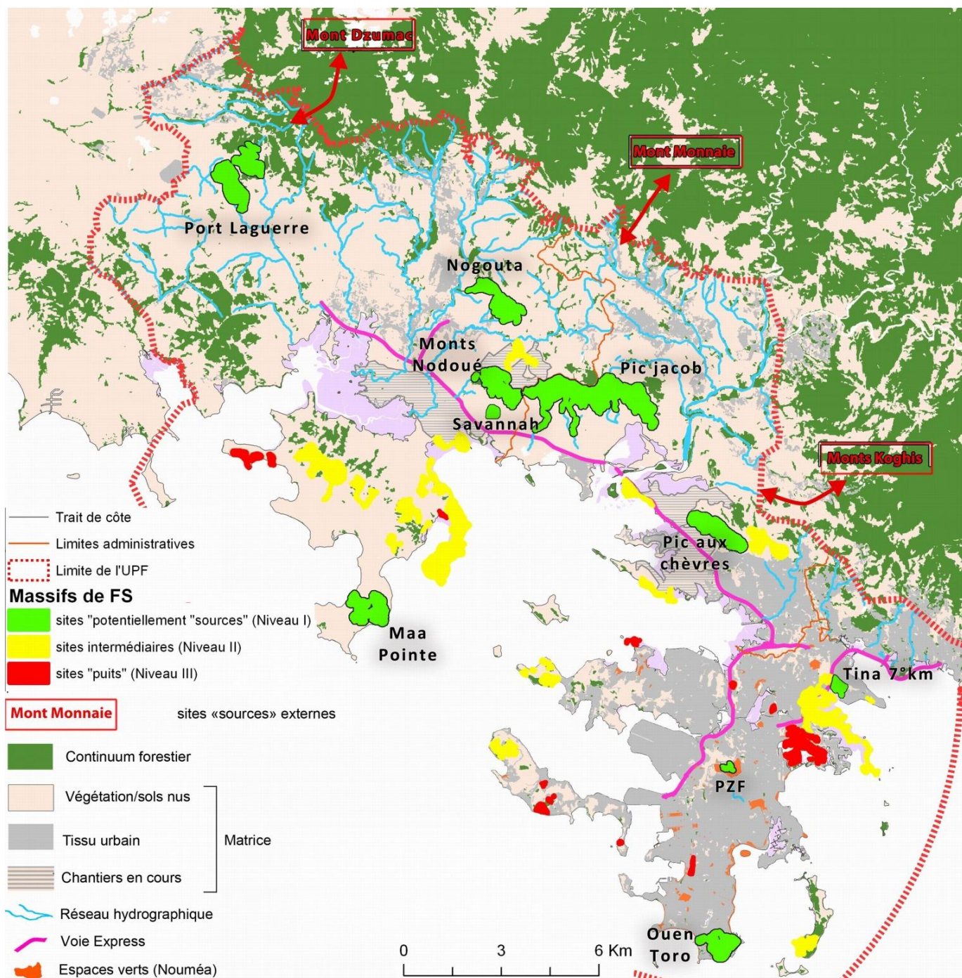
Fig. 18 : Carte des zones sources in-situ et ex-situ de l'UPF1
