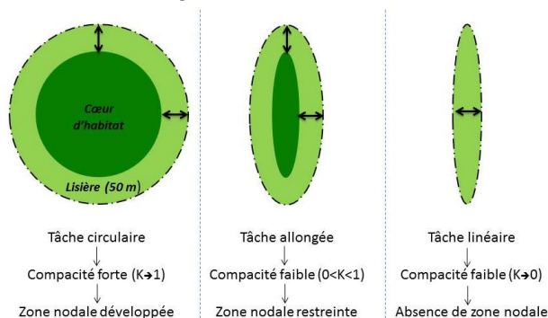
Fig. 9 : L'influence de la forme d'un massif sur la surface de la zone
