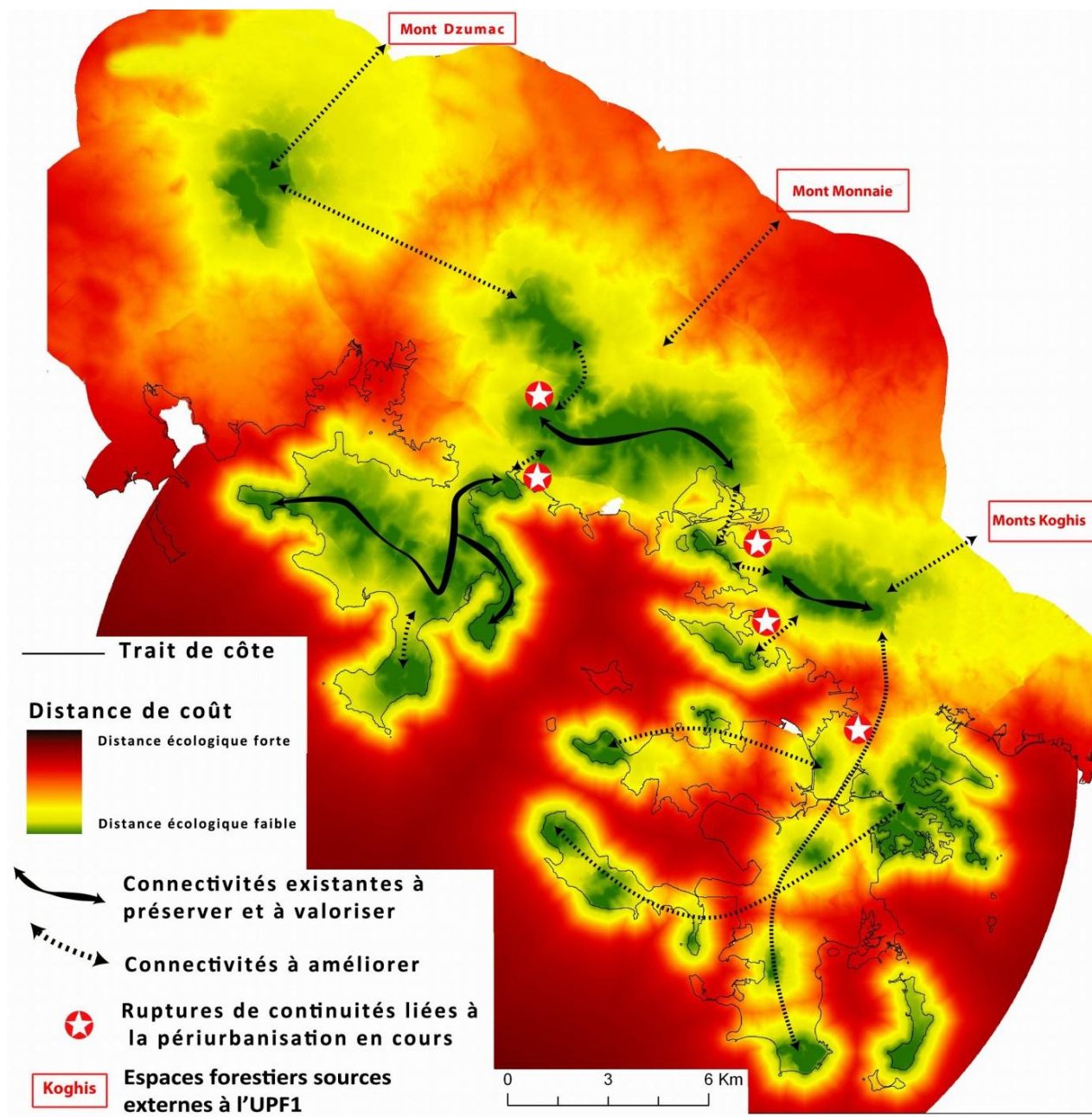
Fig. 19 : Estimation de la connectivité fonctionnelle de l'UPF 1 (Les valeurs de coût forment des anneaux concentriques écologiquement équidistants autour de la même source).
