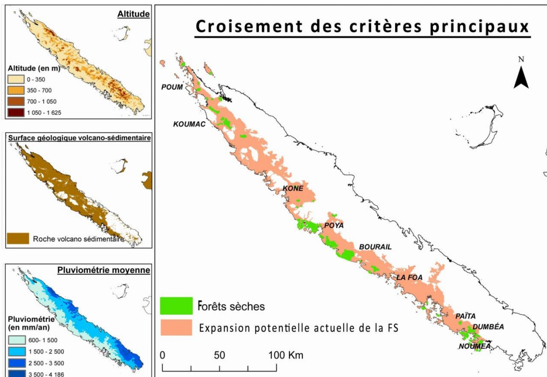
Fig. 6 : Détermination de l'aire actuelle d'expansion potentielle de la FS (données DTSI, DIMENC, METEO FRANCE)
