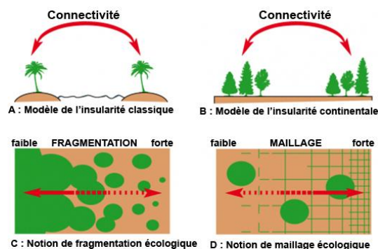
Fig. 5 : Fragmentation et connectivité en biogéographie « insulaire » (Blondel, 1995).
