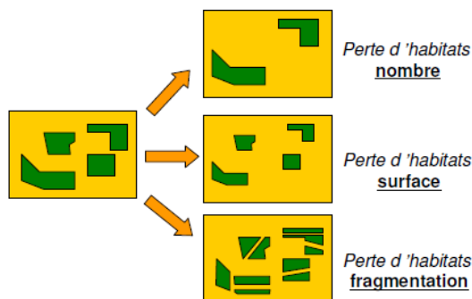
Fig. 4 : Perte d'habitats et fragmentation dans un paysage (Daniel, 2012)
