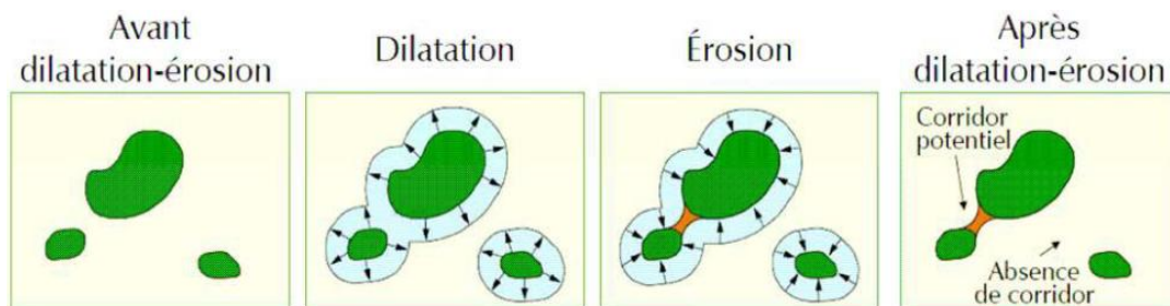
Fig. 11 : Technique de « dilatation-érosion » (d'après le Guide méthodologique trame verte et bleue – COMOP, 2009)
