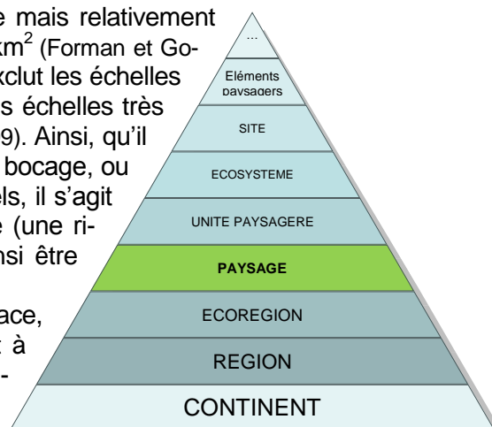
Fig. 2 : Représentation schématique des diverses échelles
