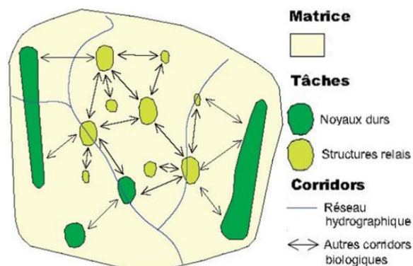
Fig. 3 : Schéma fonctionnel des trois éléments du paysage (d'après DREAL Nord-Pas-de-Calais, 2011)
