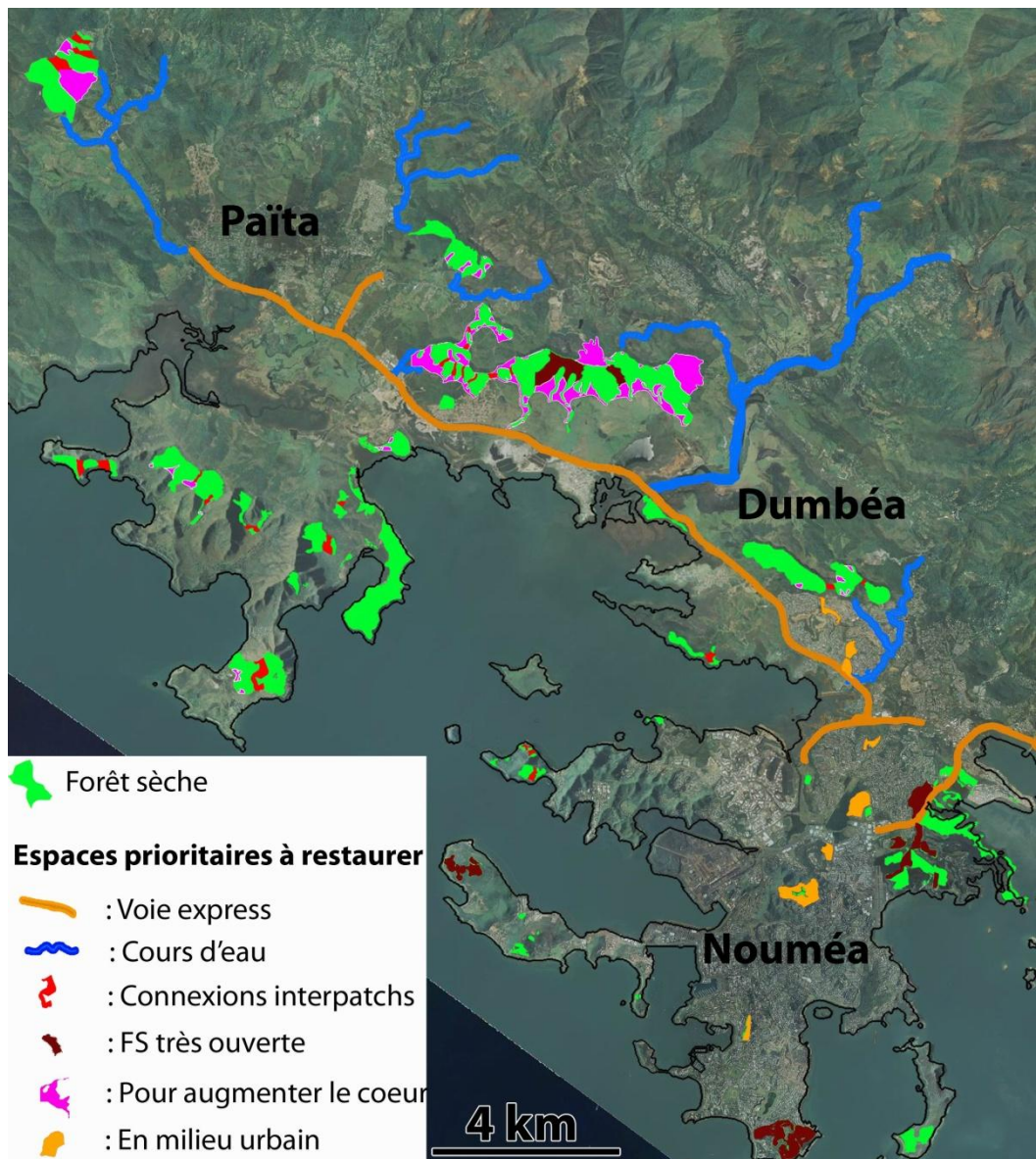
Fig. 26 : Propositions d'espaces prioritaires à restaurer dans l'UPF1
