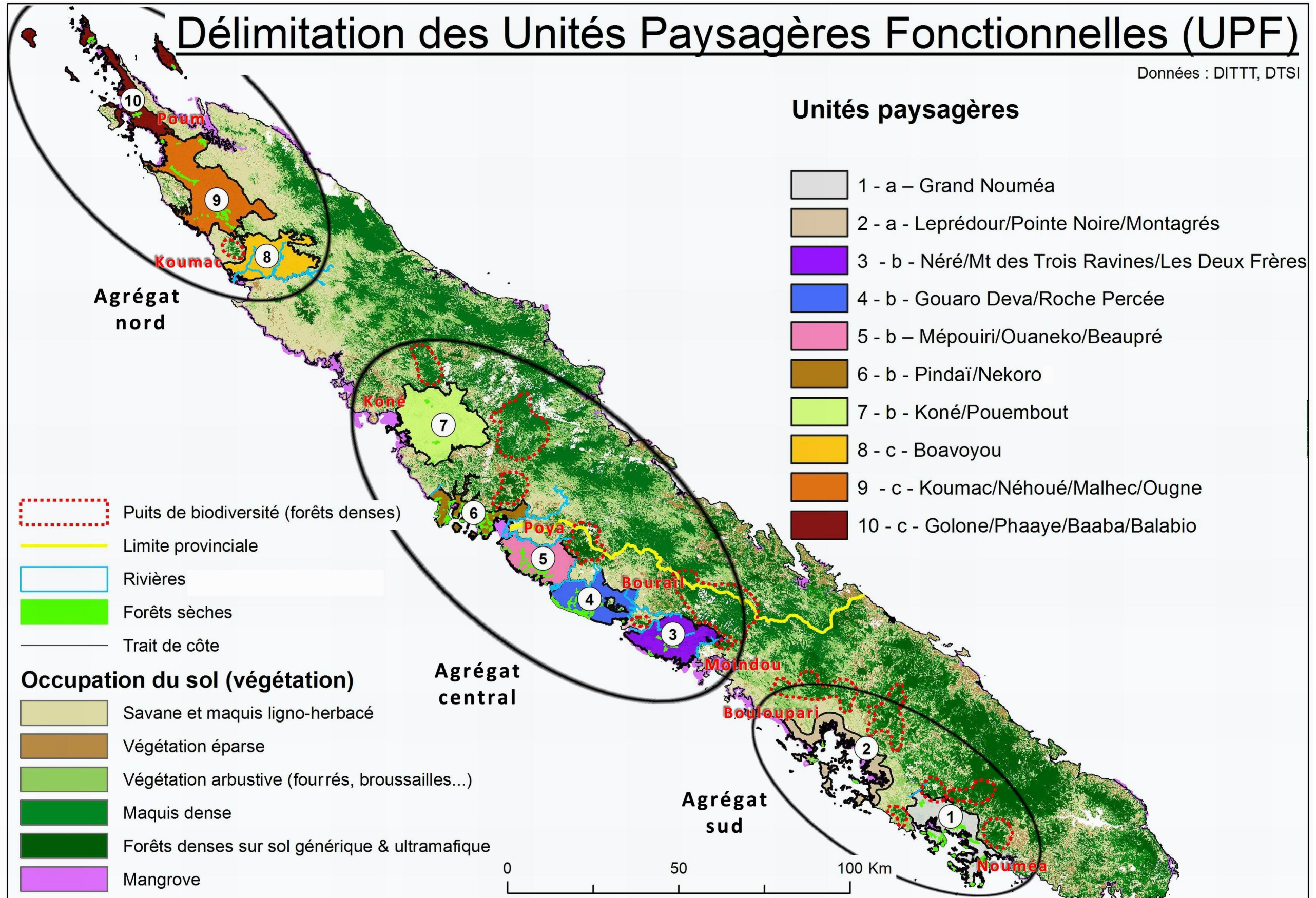
Fig. 8 : Cartographie des UPF en Nouvelle-Calédonie
