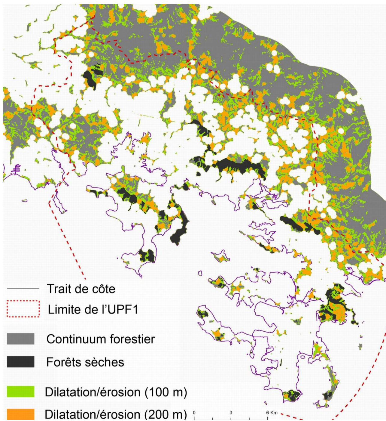
Fig. 20 : Connexions potentielles à travers la trame forestière de l'UPF1
