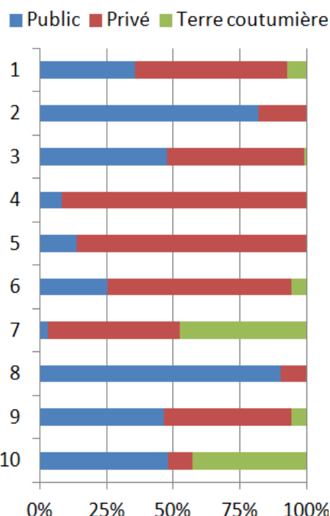
Fig. 7 : Répartition du foncier occupé par les massifs de FS dans les différentes UPF
