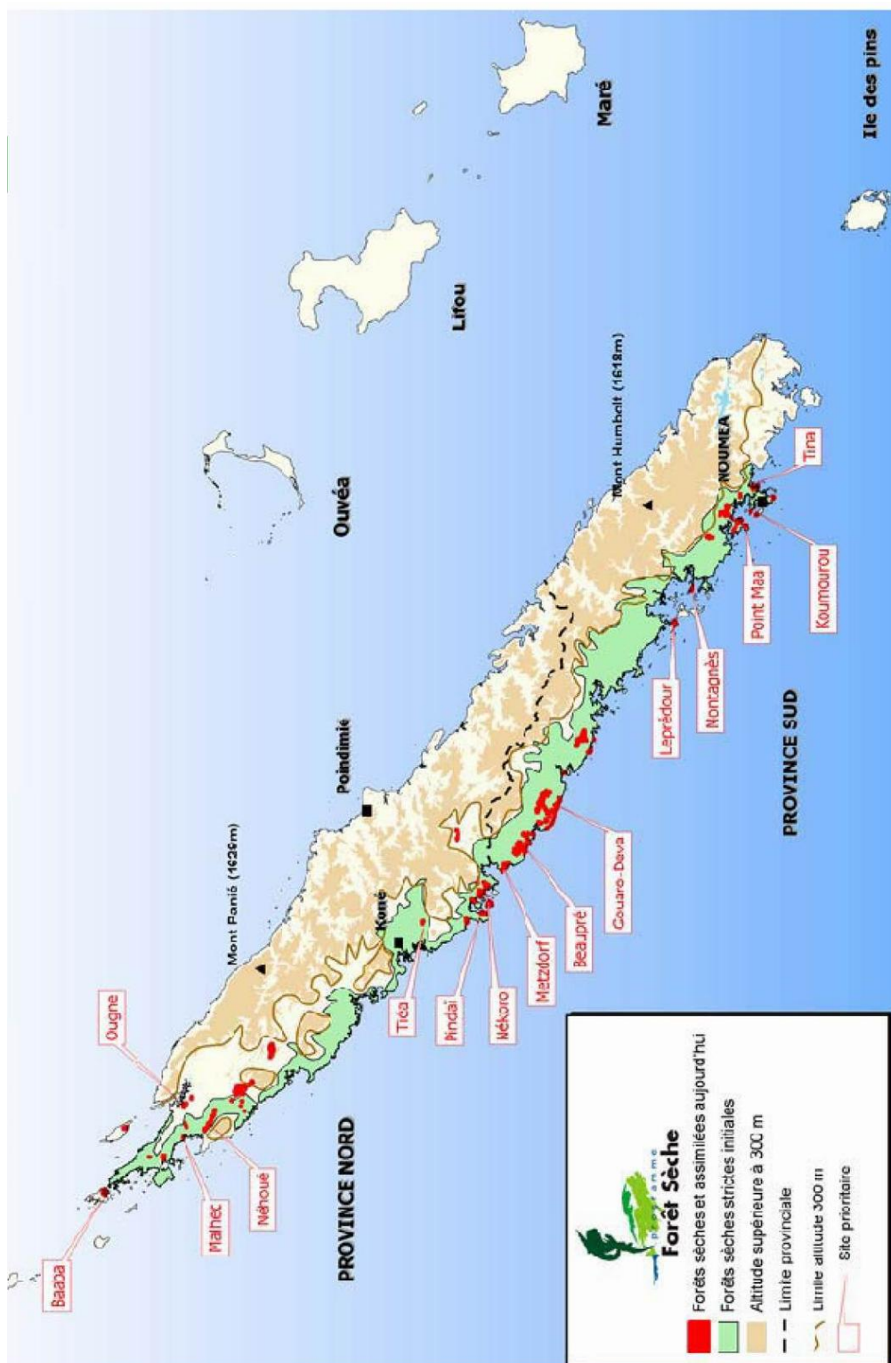
Annexe III : Première carte situant les sites des forêts sèches prioritaires du Programme Forêt Sèche (d'après Boyeau, 2001)
