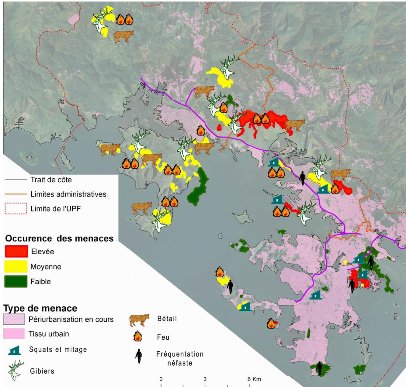
Fig. 17 : Carte des menaces recensées pour l'UPF 1 : les massifs apparaissent en jaune, rouge ou vert selon l'occurrence des menaces qui les concernent. (Remarque : Faut de cartographie générale existante (celle élaborée par l'IRD illustre la répartition des EEE autour des axes routiers), les EEE ne sont pas représentées sur la carte).
