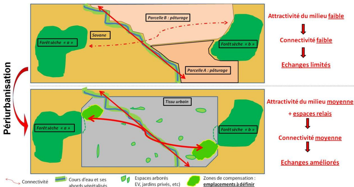
Fig. 23 : Schéma fonctionnel des potentialités de reconnexion grâce à la périurbanisation
