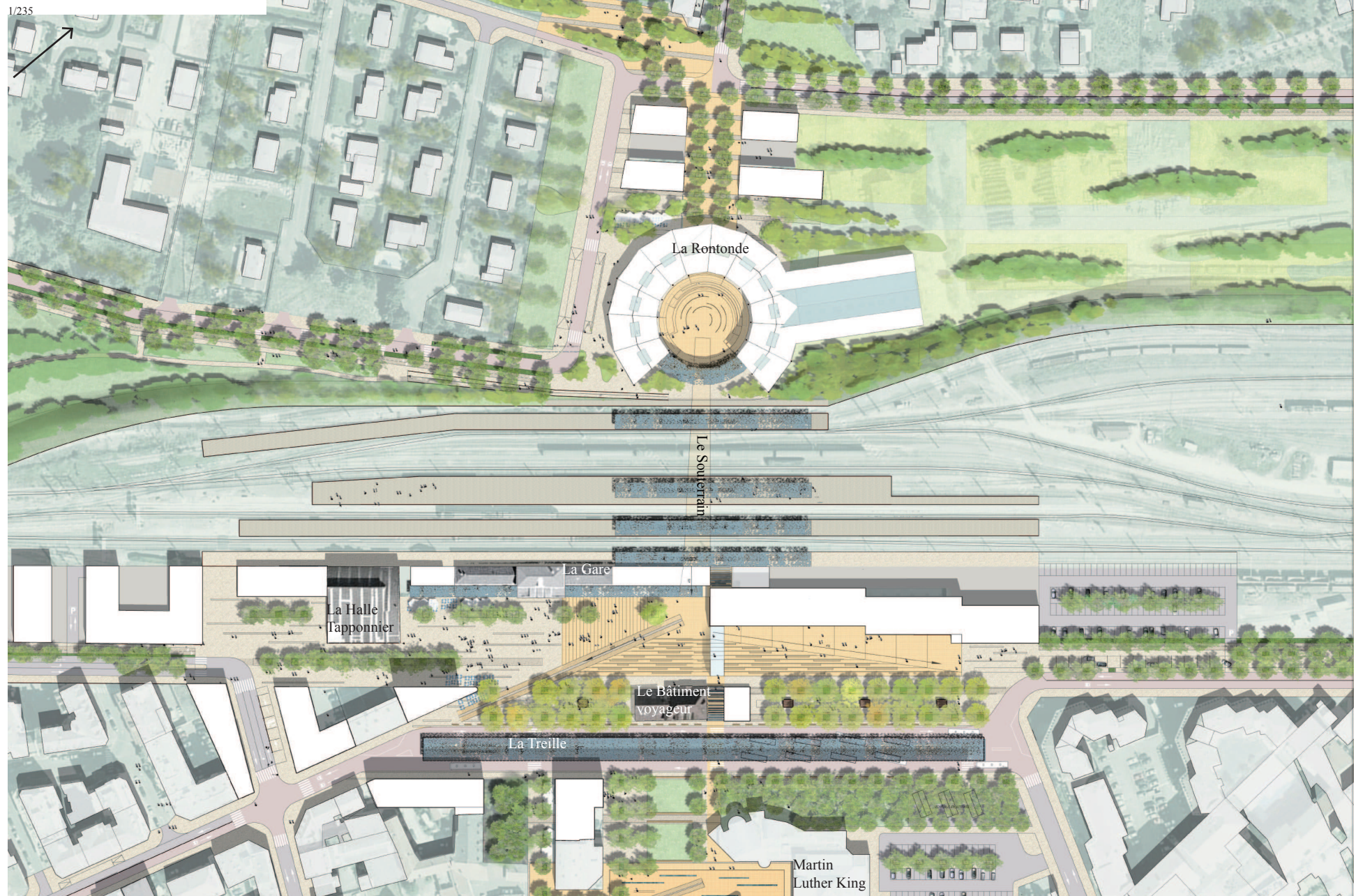
Figure 31. Plan masse du projet de pôle d'échanges de la gare d'Annemasse. Source : In Situ, 2012
