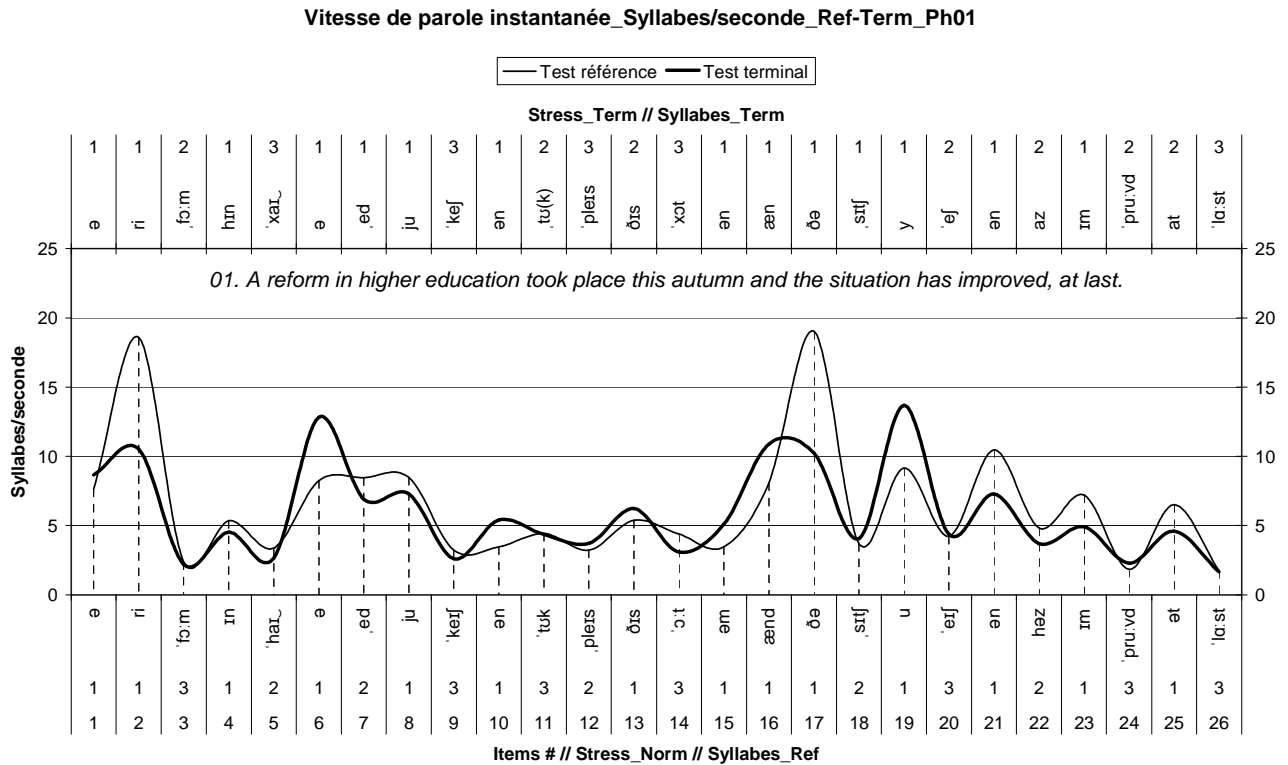
Figure 21. Vitesse de parole instantanée pour les 26 syllabes de Ph01, en T term et T ref .
