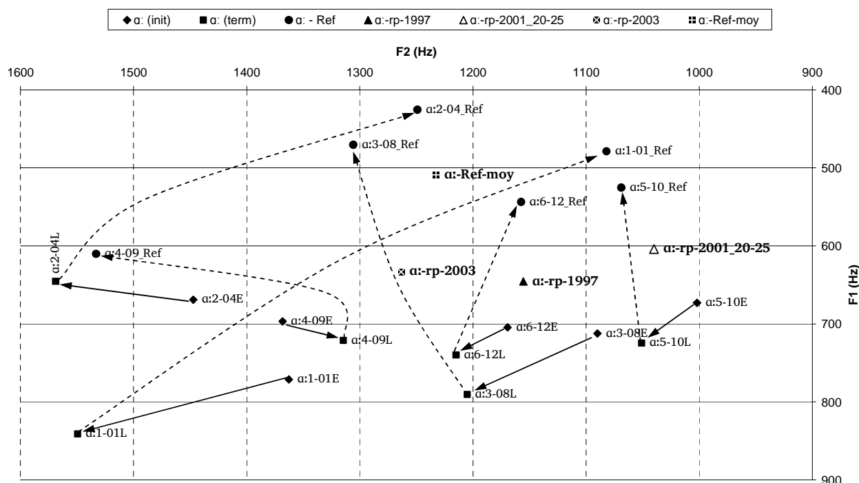
Figure 51. Valeurs mesurées de F_1 et F_2 du son /a:/ en 6 occurrences parmi les phrases Ph01 à Ph12, dans les deux versions du test T_{init} et T_{term} , les trois séries RP ( rp-1997 ; rp-2001-20-25 ; rp-2003 ) et la moyenne des données de T_{ref} ( Ref-moy ). Légendes : idem graphique précédent.
