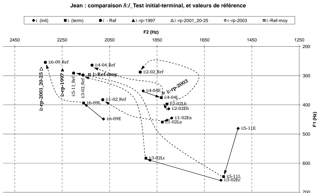
Figure 50. Valeurs mesurées de F 1 et F 2 du son /i:/ en 6 occurrences parmi les phrases Ph01 à Ph12, dans les deux versions du test T init et T term . Également : les valeurs moyennes de F 1 et F 2 des trois séries RP ( rp-1997 ; rp-2001-20-25 ; rp-2003 ) et la moyenne des données de T ref ( Ref-moy ). Les flèches pleines indiquent la variation entre T init (◆) et T term (■). Les flèches en pointillé indiquent la distance entre T term (■) et T ref (●) pour chaque occurrence. Légende identique dans les graphiques suivants.
