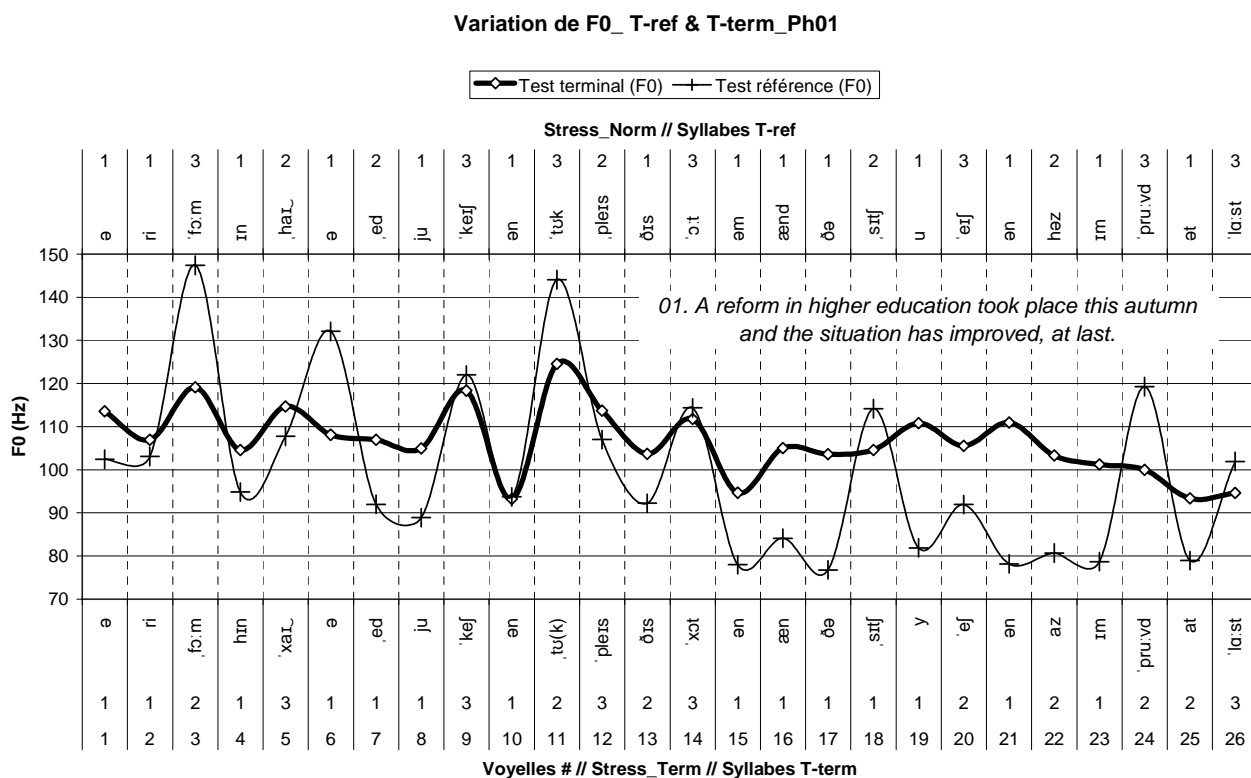
Figure 27. Evolution de F0 pour les 26 voyelles de Ph01 en T_{term} et T_{ref} .
