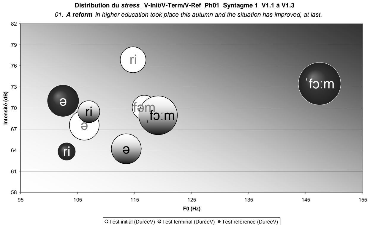
Figure 36 bis. Distribution du stress pour le syntagme #1 de Ph01 en T_{init} , T_{term} et T_{ref} . Agrandissement.
