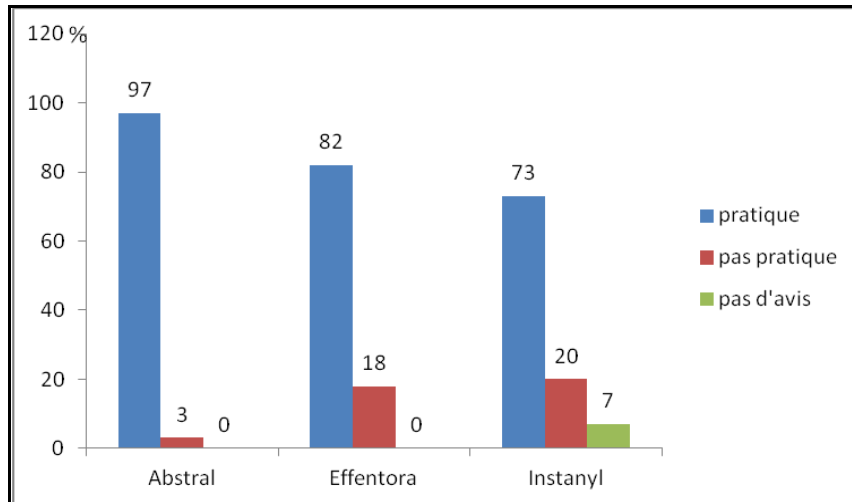
Figure 15- Opinion des patients sur la praticité globale de chaque forme
