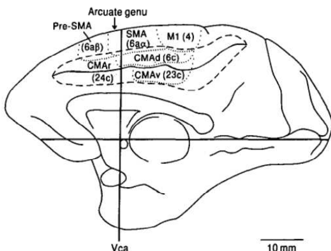
Figure 1. Organisation schématique de l'aire motrice supplémentaire et du girus cingulaire moteur d'après picard et Strick (1996). La pré-AMS et le cortex cingulaire moteur rostral sont situés en avant de la commissure antérieure. L'AMS et le cortex cingulaire moteur ventral et dorsal sont situés en arrière de la commissure antérieure dans le plan CACP.
