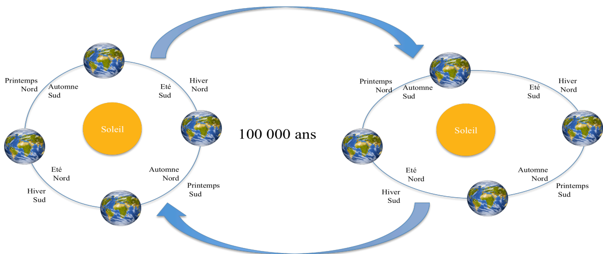
Figure 2. Excentricité de l'orbite terrestre
