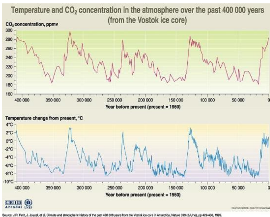
Figure 16. Teneur en CO 2 des carottes glaciaires antarctiques. (14)
