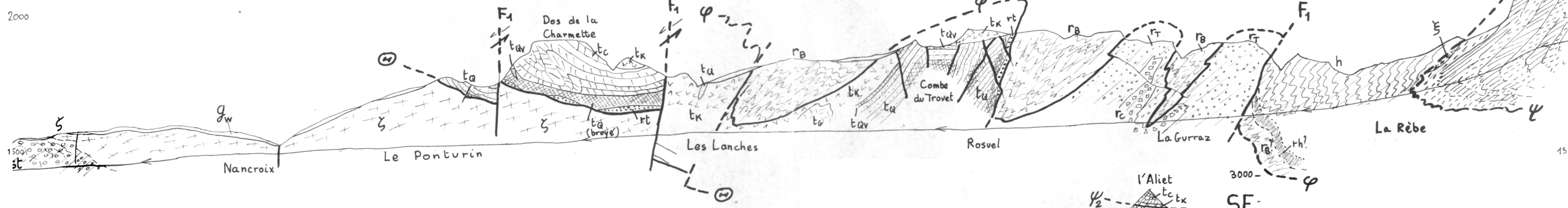
COUPE BB
