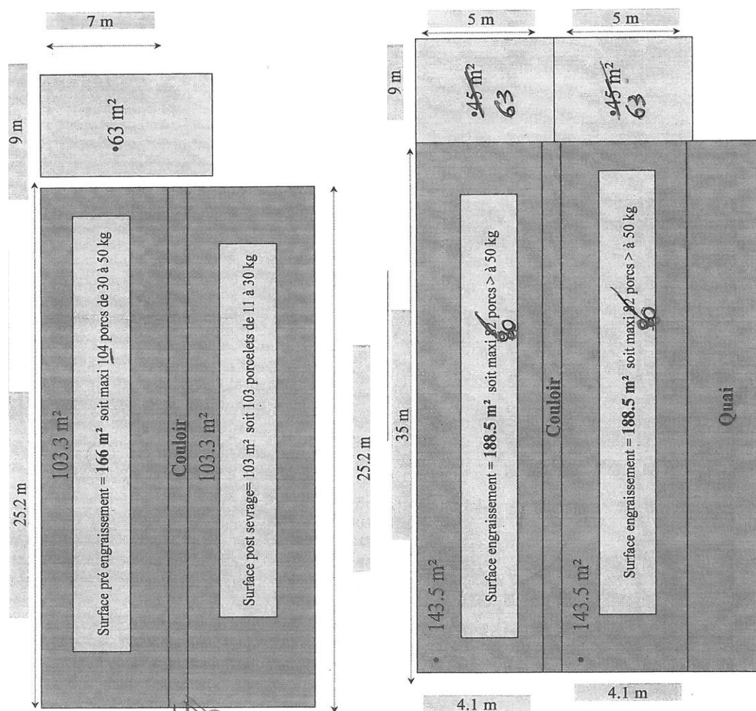
Ci-dessus : A gauche, plan du bâtiment mixte post-sevrage/pré-engraissement; à droite, plan du bâtiment d'engraissement
