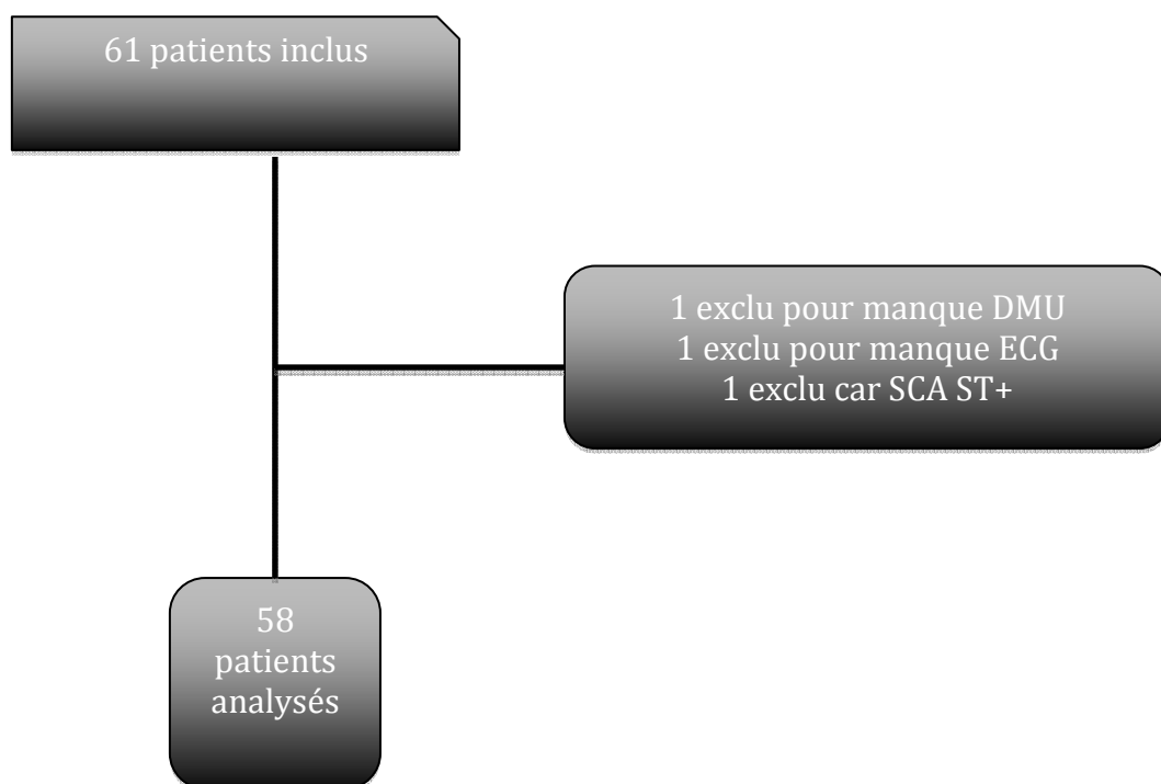
Figure 1. Diagramme d'inclusion
