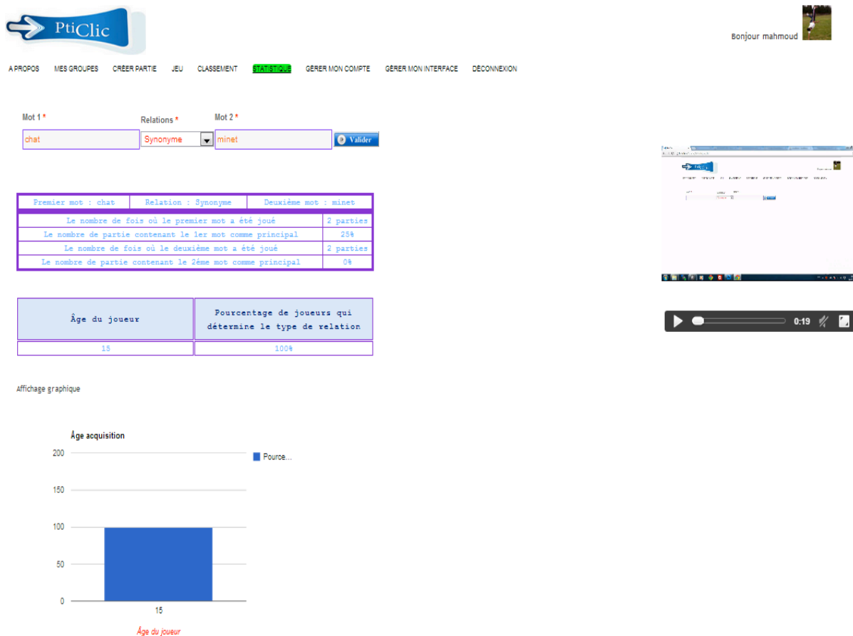
Figure 31 : Page Statistique
