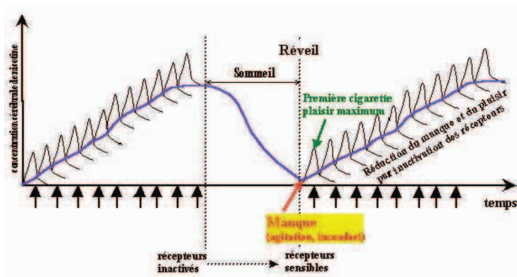
Figure 14 : La concentration de nicotine par rapport au temps.
