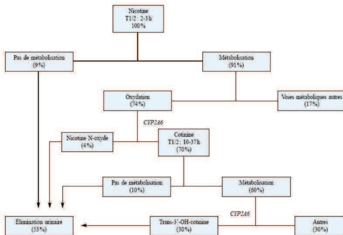
Figure 11 : Pharmacocinétique de la nicotine.
