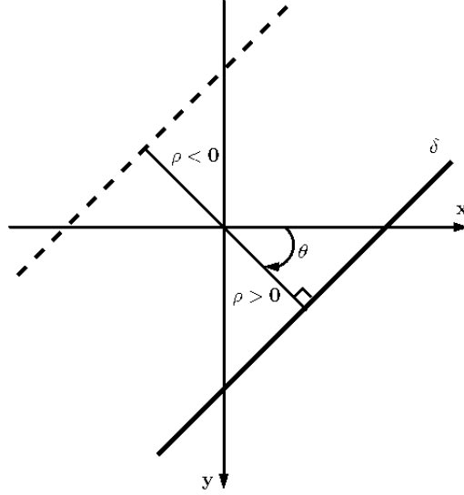
FIGURE 4.4 – Représentation d'un ligne en (\rho, \theta)
