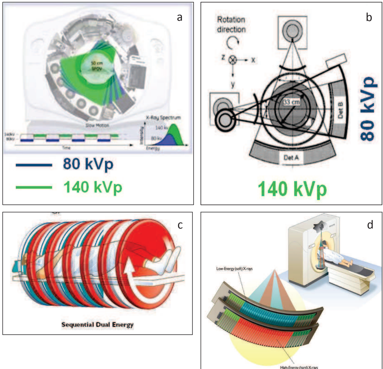
Figure 15: Approches technologiques du scanner double énergie.
