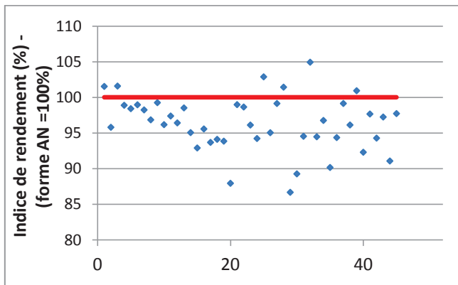
Figure 19 : Indices de rendement pour la forme urée, sans augmentation de dose - Effet système
