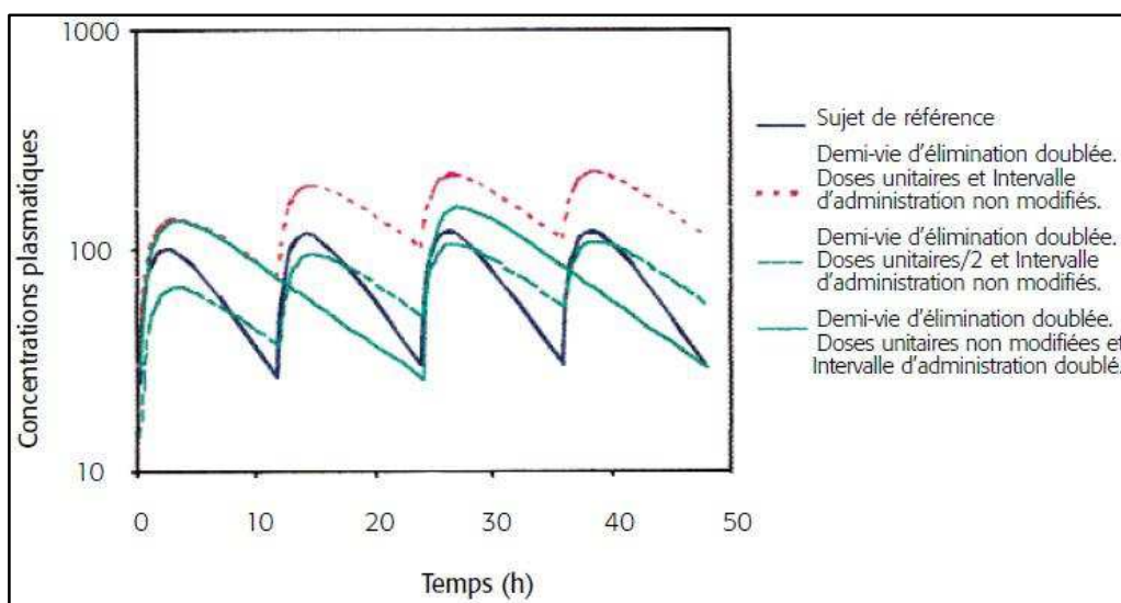
Figure 18 : Effets pharmacocinétiques selon des modifications posologiques
